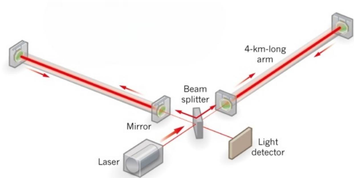
Figura 2.3: Esquema básico de un interferómetro de tipo Michelson operado por la colaboración LIGO. La perturbación métrica transversal induce una variación diferencial en los brazos, revelando la onda gravitacional a través de un patrón de interferencia desplazado [14].
