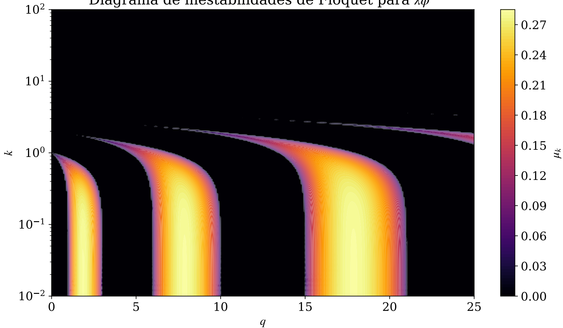
Diagrama de inestabilidades de Floquet para \lambda\phi^4
