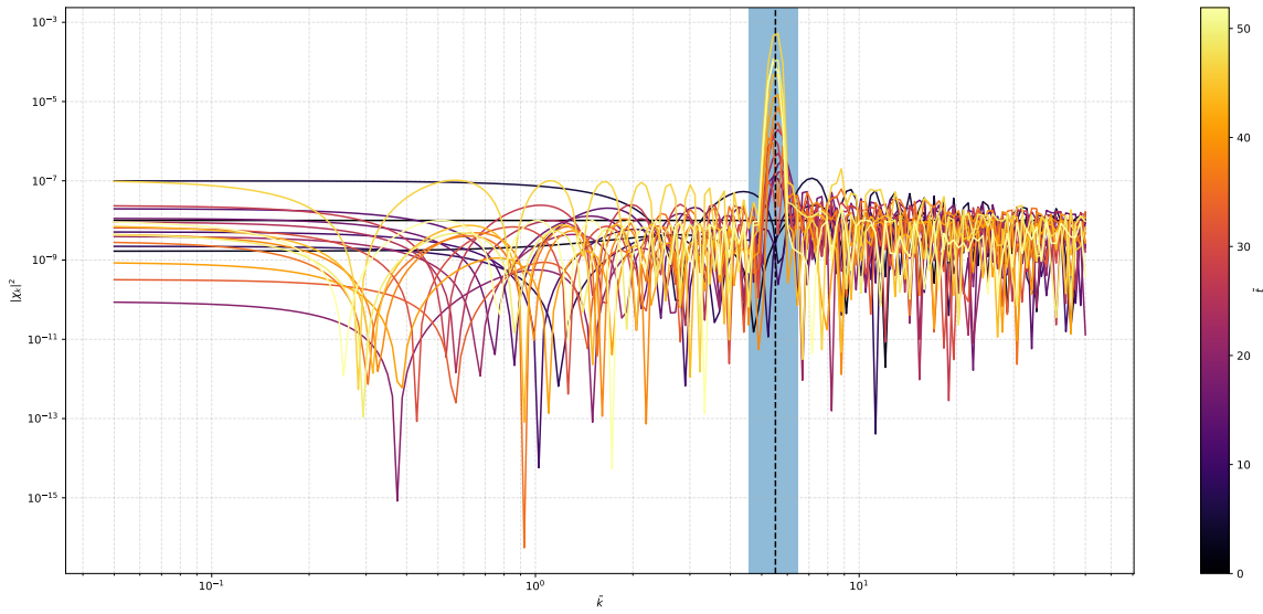
Figura 3.7: Evolución del espectro de potencias del campo hijo \mathcal{P}_\chi(k, \tau) . Se sombrea en azul la banda de resonancia calculada a partir del análisis de Floquet. Se observa que el espectro se amplifica en la banda de resonancia teniendo el máximo ubicado en el punto donde este coeficiente es máximo.
