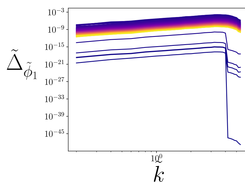
Dinámica del campo hijo utilizando un modelo m^2\phi^2
