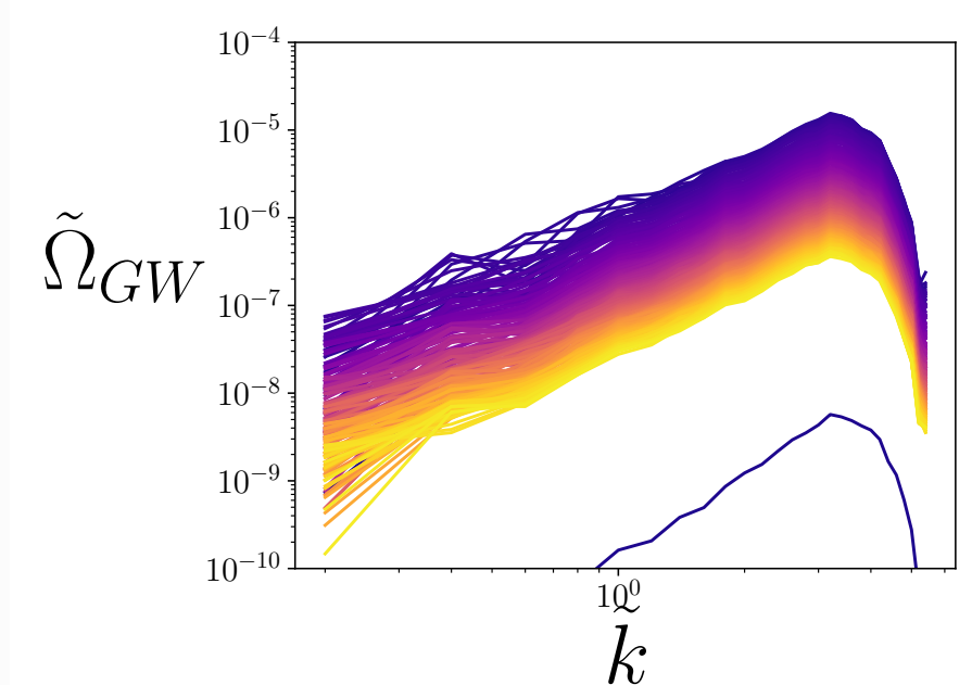
Espectro de GW hoy utilizando un modelo m^2\phi^2
