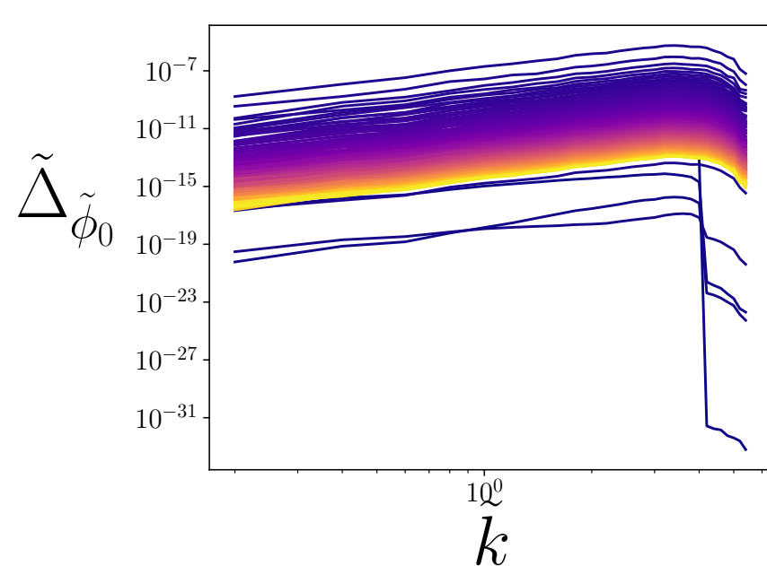
Dinámica del campo inflatón utilizando un modelo m^2\phi^2
