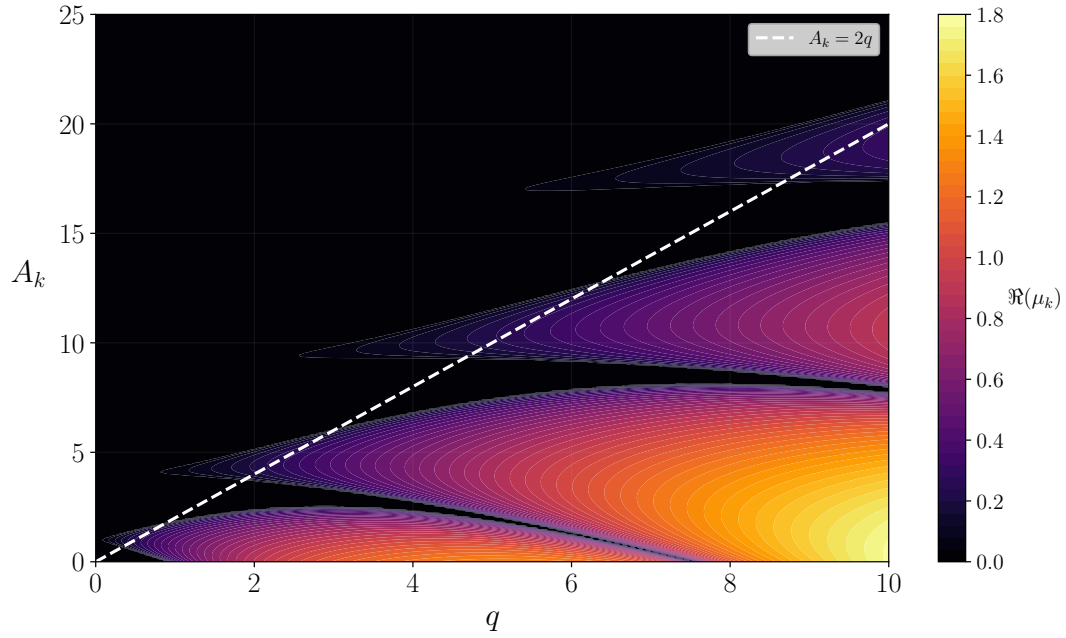
(a) m^2\phi^2
