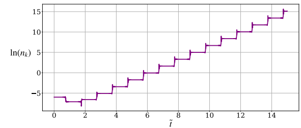
Figura 22: número de partículas para broad resonance. Para esta figura tomamos q = 200 y A_k = 401 .
