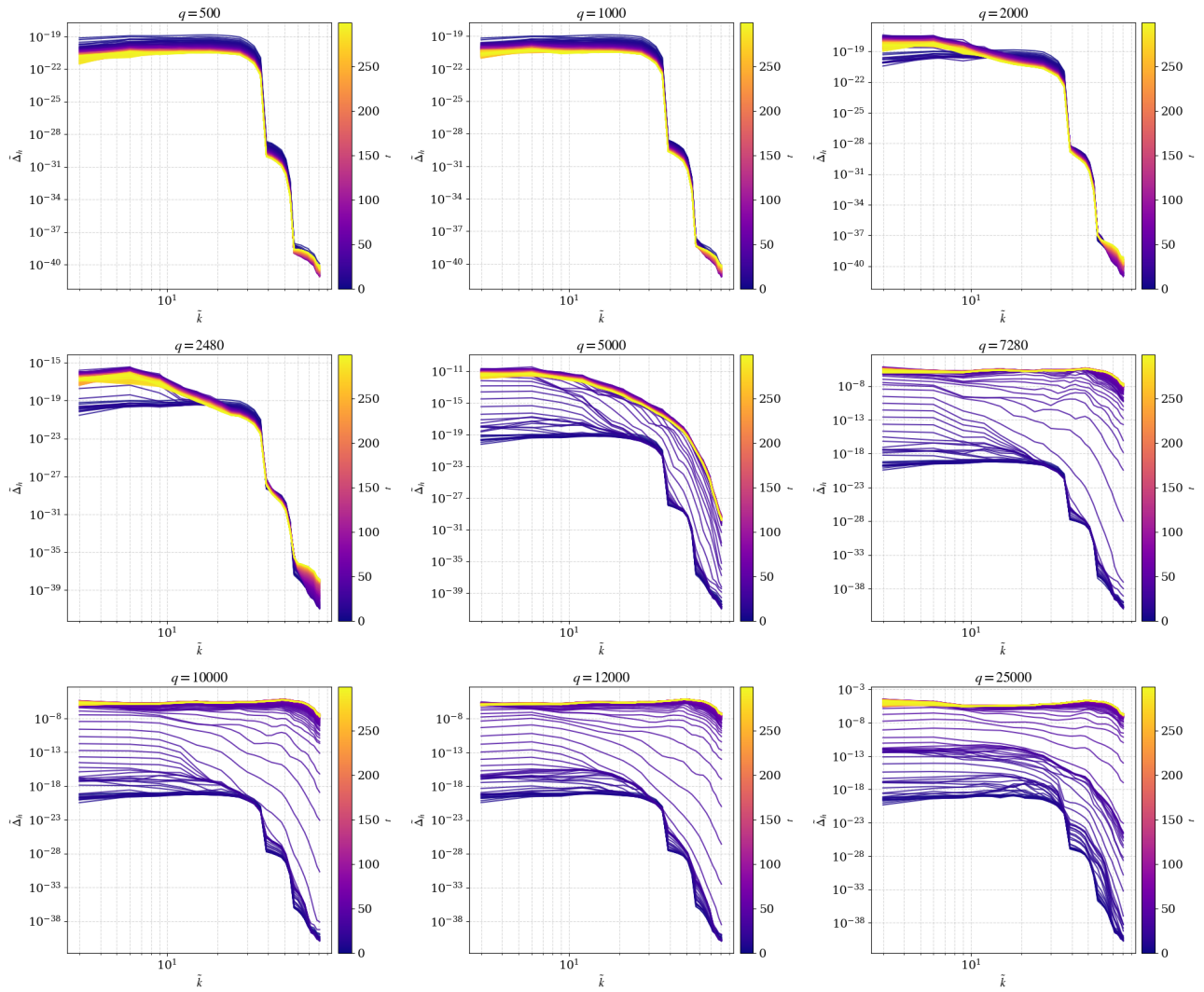
Figura 13: espectro de potencia para las ondas gravitacionales en un modelo de tipo m^2\phi^2 .
