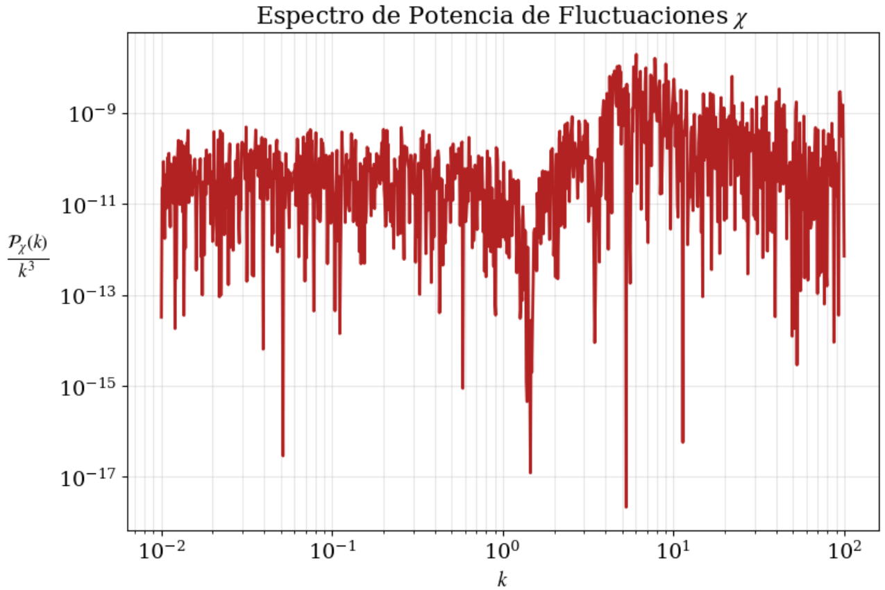
Figura 33: espectro de potencias lineal para las fluctuaciones del campo hijo.
