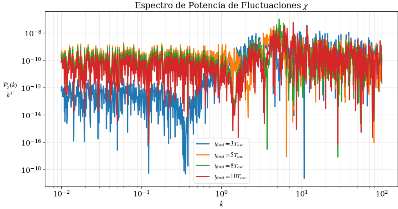
Figura 34: espectro de potencias lineal para las fluctuaciones del campo hijo para distintos tiempos.
