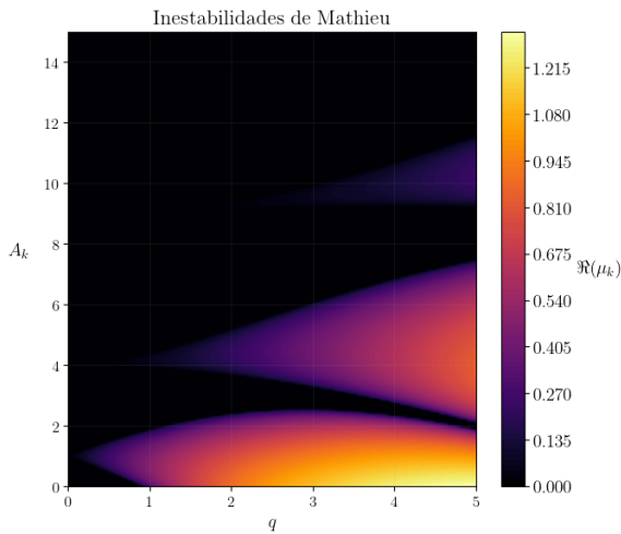
Figura 15: en esta imagen podemos ver cómo son las bandas para valores de q entre 0 y 5, y valores de A_k entre 0 y 15. Esta imagen es la misma que aparece en el texto de Mishra.
