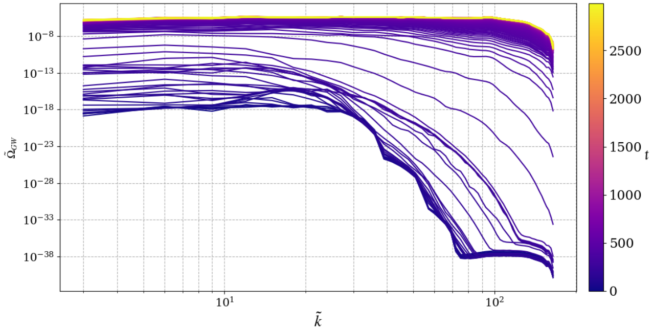
Figura 9: espectro de potencia para las ondas gravitacionales en un modelo de tipo Starobinsky para q = 4 \times 10^4 .
