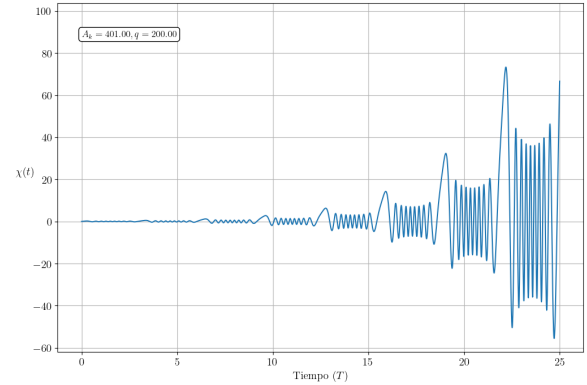
Figura 20: en esta imagen tenemos la evolución del modo con q = 200 y A_k = 401 lo que nos da una narrow resonance
