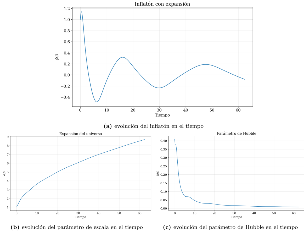
Figura 30: evolución del background para el modelo \lambda\phi^4 .
