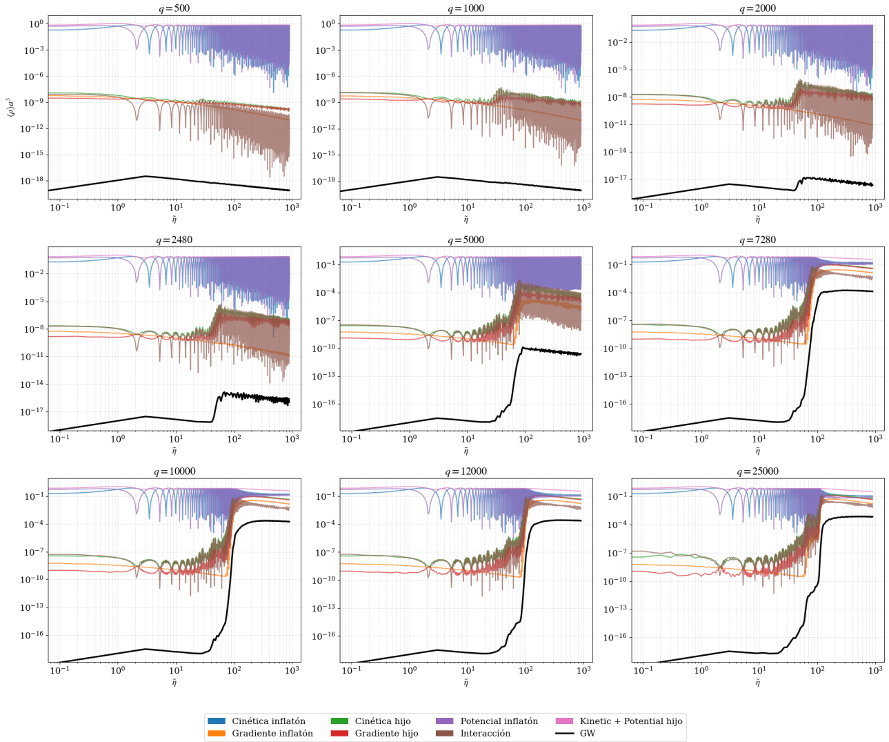
Figura 14: evolución de las densidades de energía de cada tipo y ondas gravitacionales.
