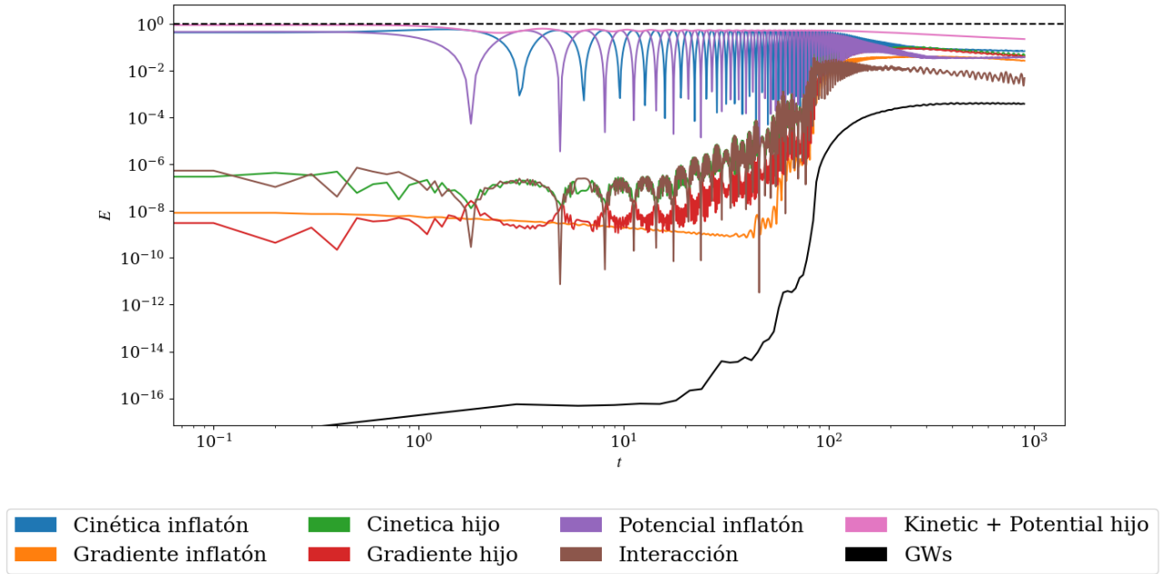
Figura 8: evolución en la densidad de energía de cada término de la acción y energía de las ondas gravitacionales en el tiempo en un modelo de tipo Starobinsky para q = 4 \times 10^4 .
