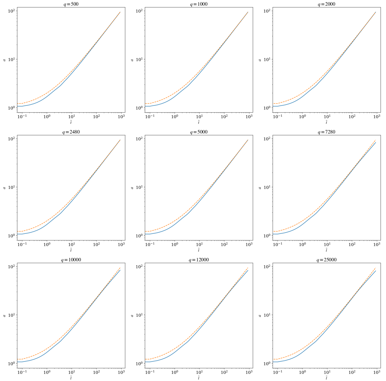
Figura 10: evolución de a(t) para el potencial m^2\phi^2 , podemos ver que a \sim t^{2/3} .
