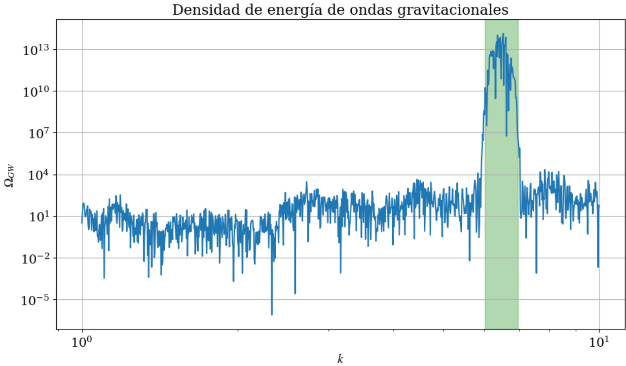
Figura 29: distribución en k para la densidad de energía de ondas.
