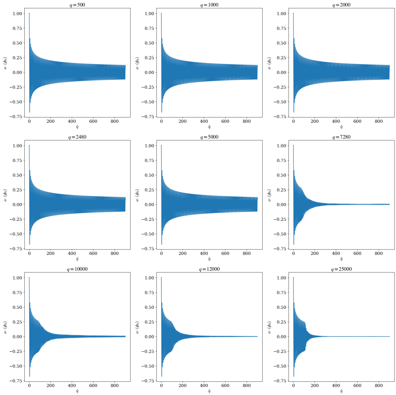
Figura 11: evolución de \phi(t) para el modelo m^2\phi^2 .
