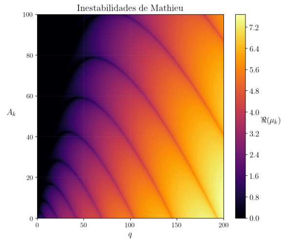
Figura 16: en esta imagen podemos ver cómo son las bandas para valores de q entre 0 y 200, y valores de A_k entre 0 y 100.
