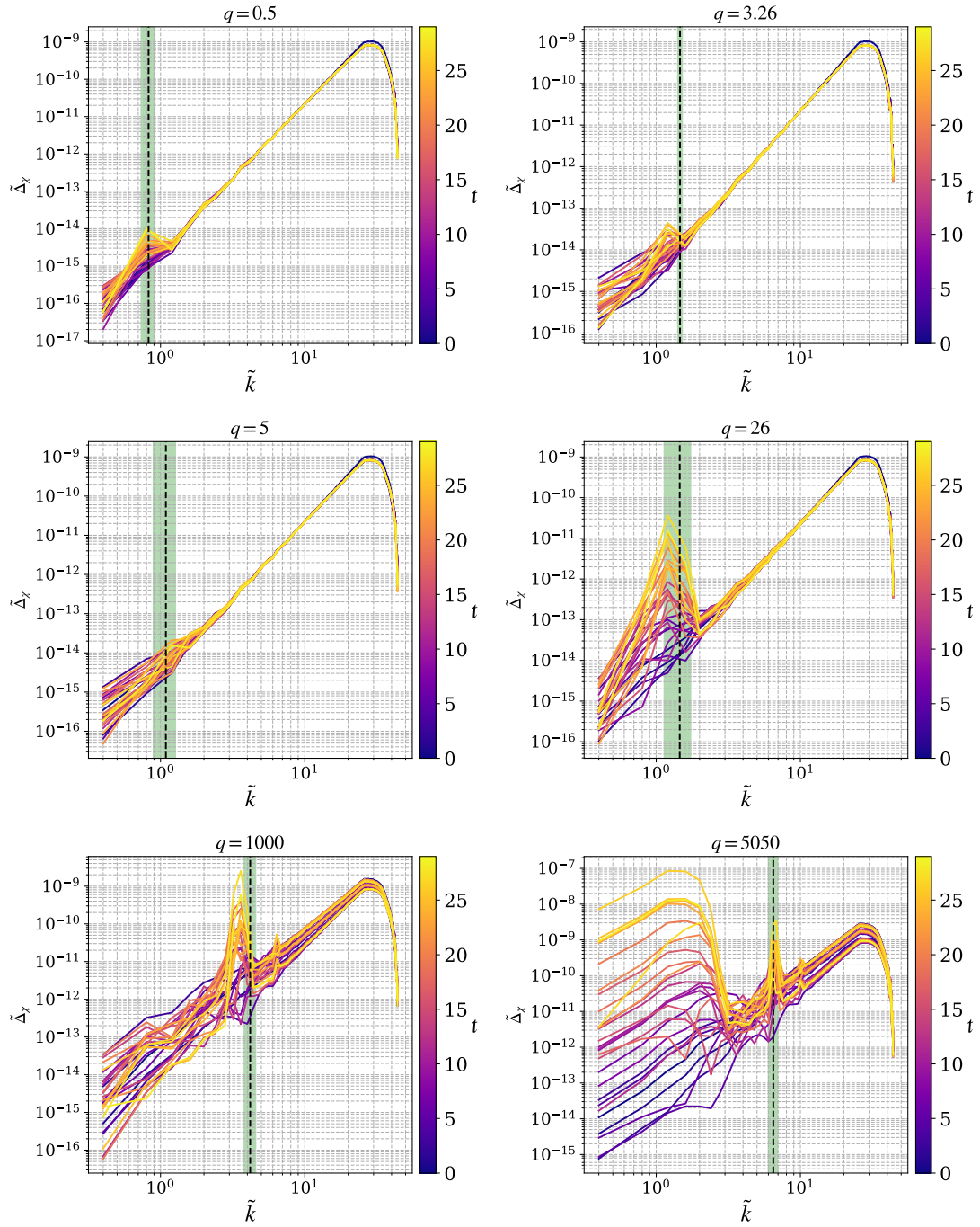
Figura 4.1: Espectro de potencias del campo hijo para distintos valores del parámetro de acoplamiento q . Se sombrea en verde la banda de frecuencias que se ve ampliada de acuerdo con el análisis de Floquet y en la misma franja se observa que se encuentra el pico principal del espectro.
