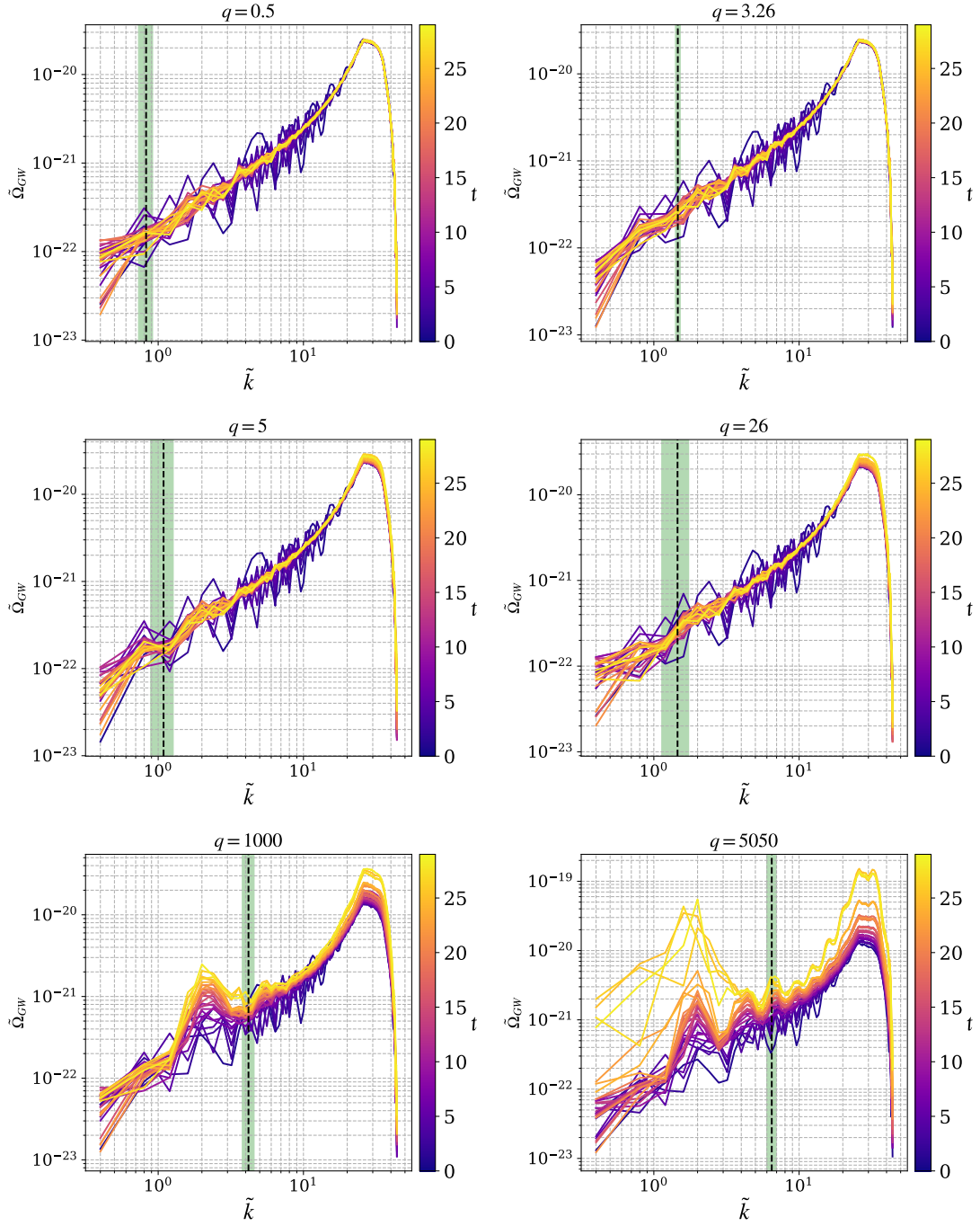
Figura 4.3: Espectro de potencias de ondas gravitacionales para distintos valores del parámetro de acoplamiento q . Se sombrea en verde la banda de frecuencias que se vé amplificada de acuerdo con el análisis de Floquet y en la misma franja se observa que se encuentra el pico principal del espectro, además se observan otros picos consecuencia de la convolución de modos.
