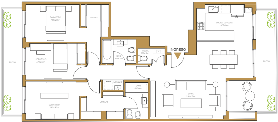
PLANTA 4 AMBIENTES
