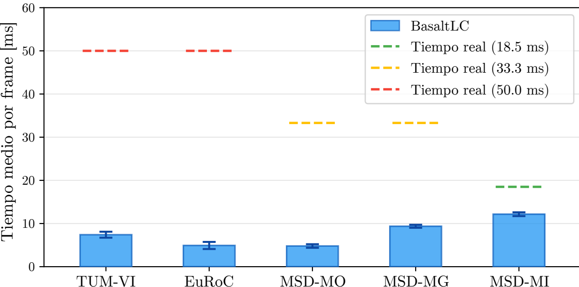
Tiempo medio de procesamiento por frame según grupo de secuencias para BasaltLC
