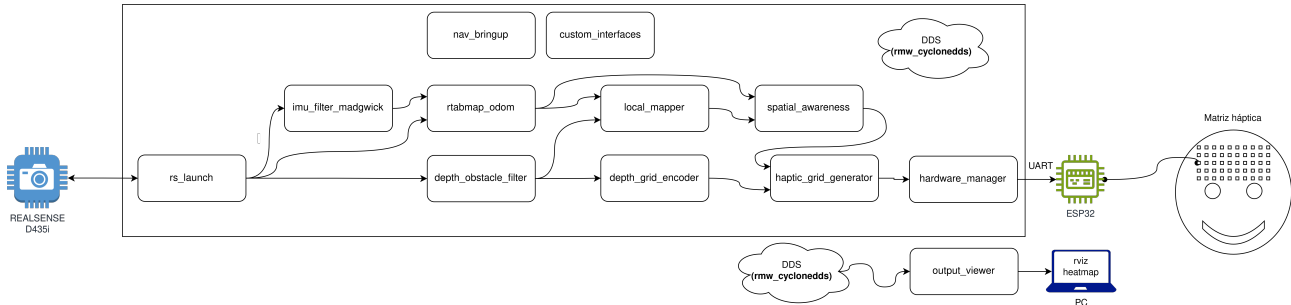
Figura 4.3: Arquitectura v2.
