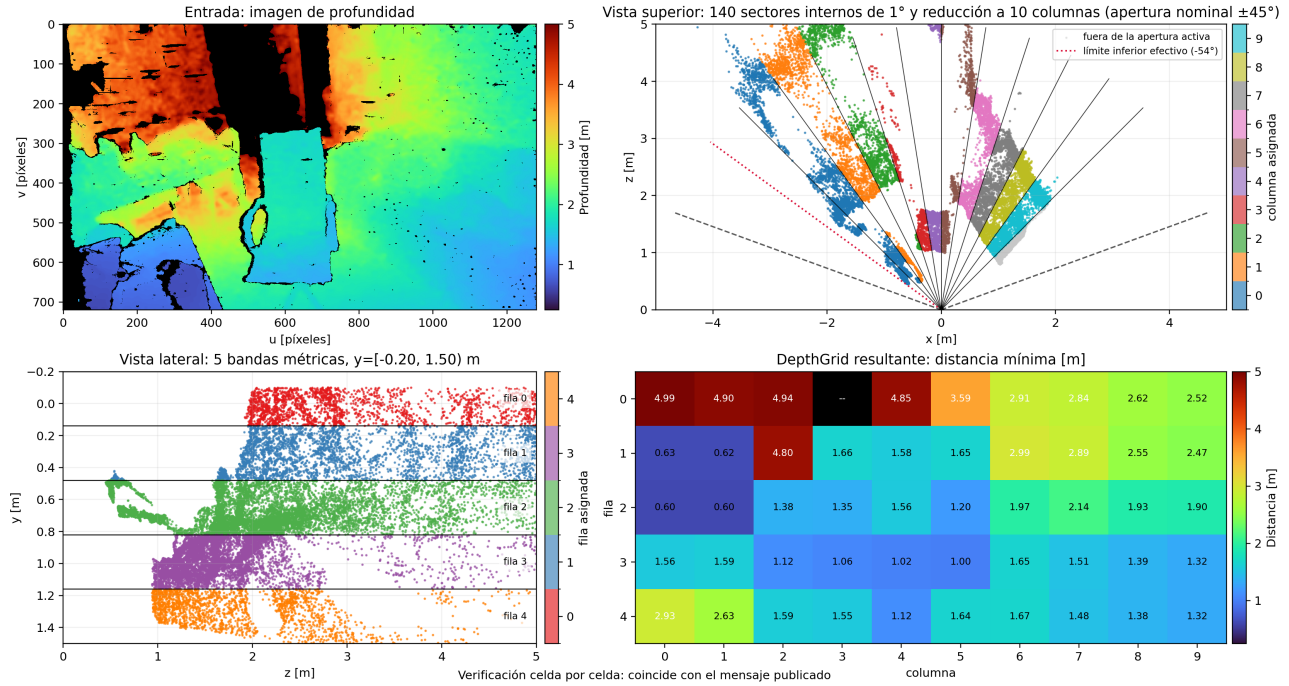
Figura 5.8: Codificación angular y vertical de una nube en una DepthGrid de 5 filas por 10 columnas.
