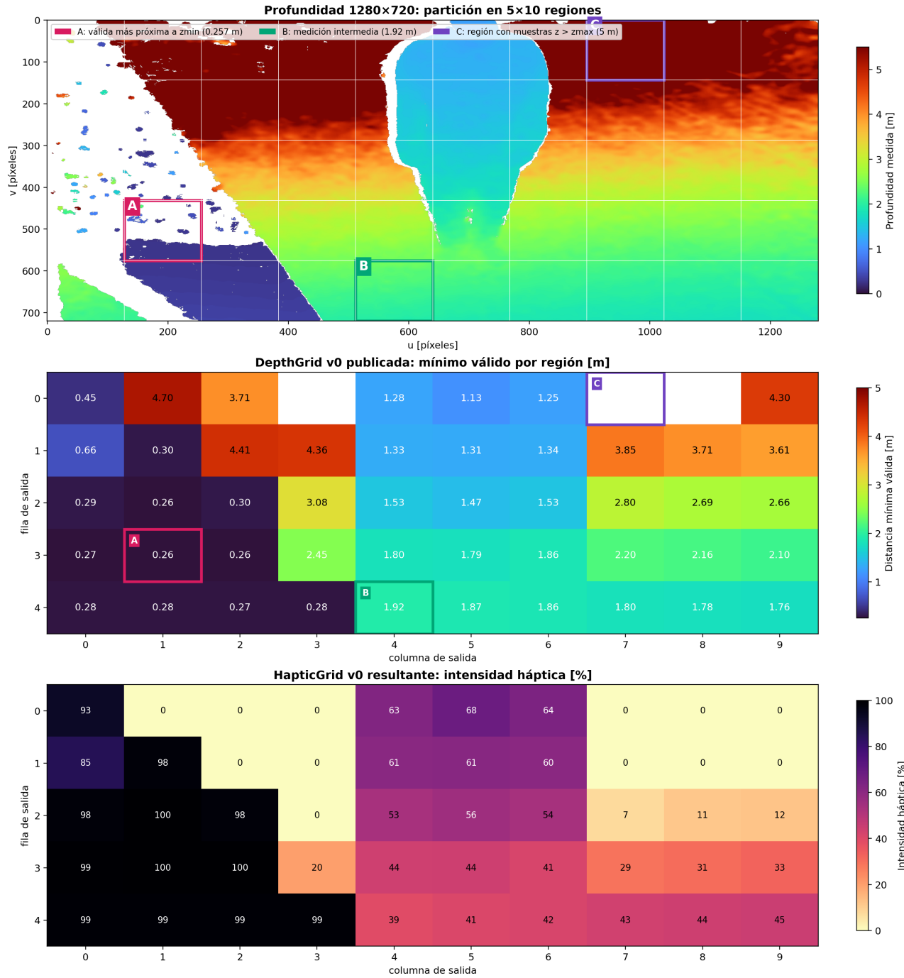
Figura 5.1: Reducción de la configuración inicial multirango E1-A a una DepthGrid de 5 \times 10 . A señala la medición válida más próxima a z_{\min} ; B, una distancia intermedia; y C, una región compuesta exclusivamente por muestras mayores que z_{\max} . v0 descarta estas últimas y publica la celda C sin evidencia. El tercer panel muestra la HapticGrid: las distancias se convierten a intensidad y las celdas que no producen estimulación se representan con valor cero.
