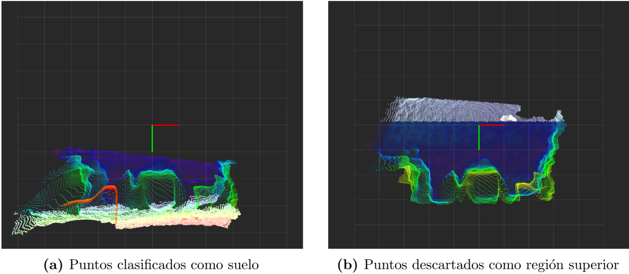
Figura 5.6: Clasificación geométrica de la nube alineada antes de construir la grilla háptica.
