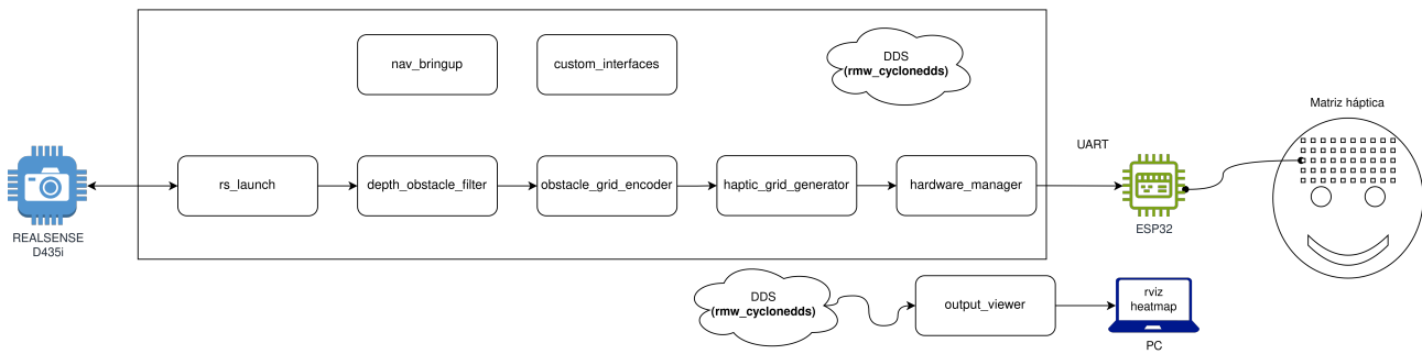
Figura 4.2: Arquitectura v1.
