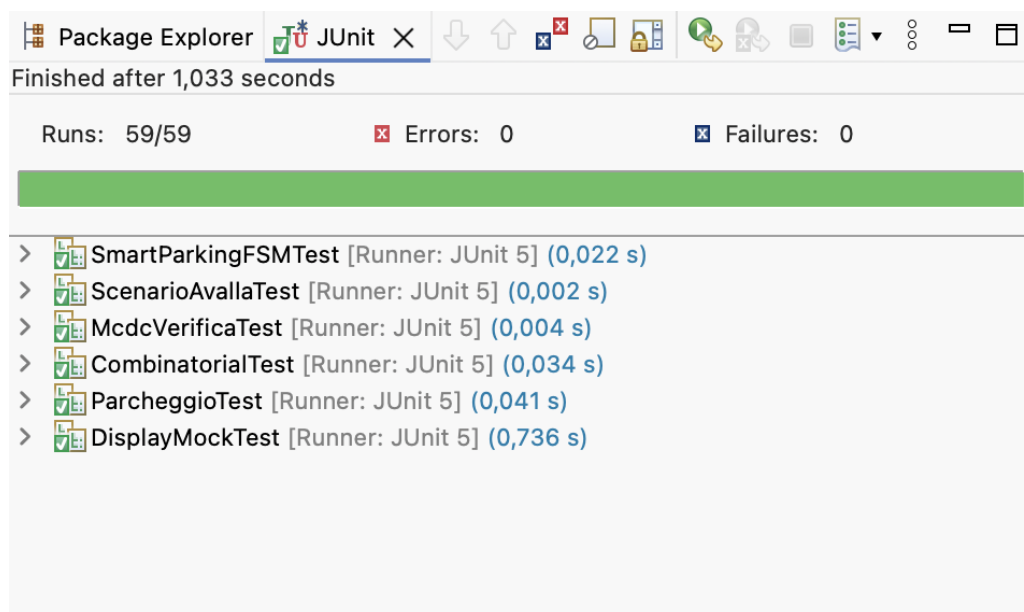
Figura 16: Esecuzione di tutta la suite JUnit
