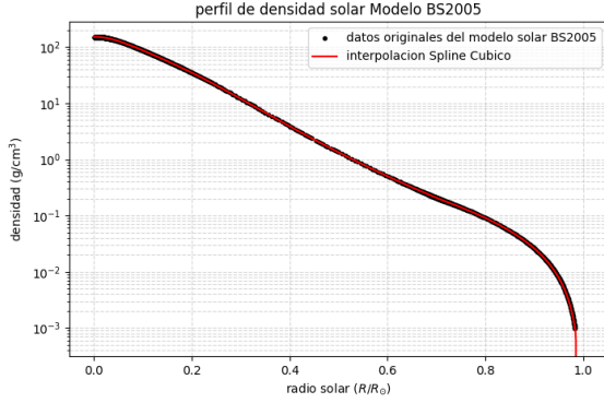
Figura 1: Perfil de densidad de masa solar construido mediante interpolación de Splines Cúbicos Naturales a partir de los datos crudos del Modelo Solar Estándar BS2005 (bs05op.dat).
