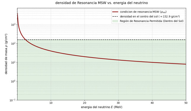
Figura 5: Densidad de resonancia teórica MSW ( \rho_{\text{res}} ) en función de la energía del neutrino. La línea horizontal marca la densidad máxima del Sol, y la región sombreada indica el dominio de resonancia físicamente accesible.
