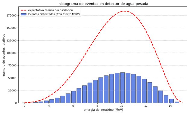
Figura 6: Histograma de eventos esperados en el detector terrestre de Agua Pesada por Corriente Cargada. Las barras azules muestran el espectro con el efecto MSW; la línea roja segmentada indica la predicción teórica sin oscilación (hipótesis nula).
