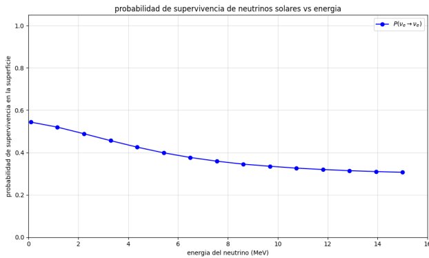
Figura 3: Probabilidad de supervivencia final del neutrino electrónico P(\nu_e \rightarrow \nu_e) medida en la superficie solar en función de su energía de emisión.
