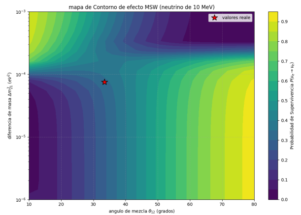
Figura 4: Mapa de contorno de la probabilidad de supervivencia P(\nu_e \rightarrow \nu_e) en el espacio de parámetros ( \theta_{12} vs \Delta m_{21}^2 ) para neutrinos de E = 10 MeV. La estrella roja marca los valores reales medidos experimentalmente.
