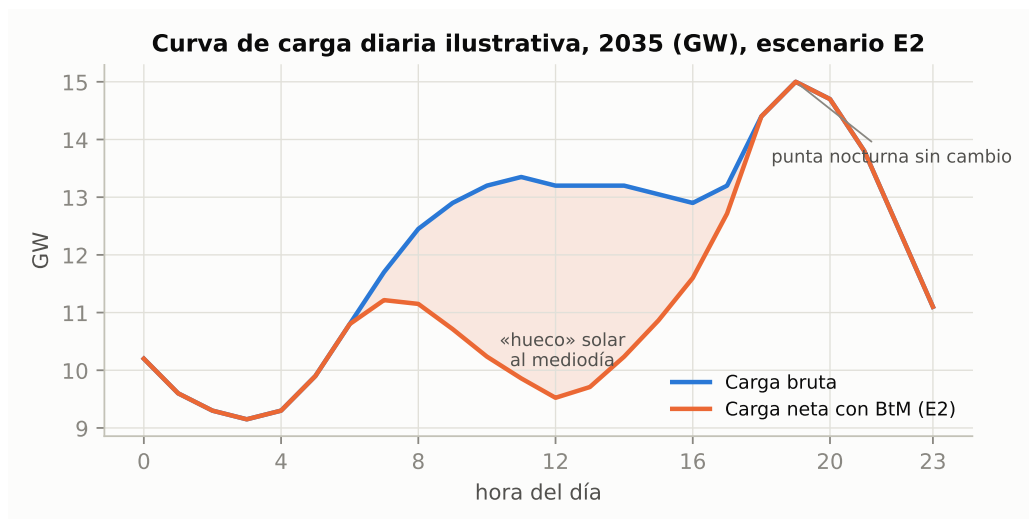
Figura A4: Curva de carga diaria ilustrativa a 2035 bajo E2 (forma típica de día hábil del SIN, punta nocturna normalizada a la potencia máxima proyectada). El BtM fotovoltaico deprime el mediodía (~3,7 GW) sin tocar la punta de las 19-20 h: el fenómeno de la “curva de pato”. Elaboración propia.
