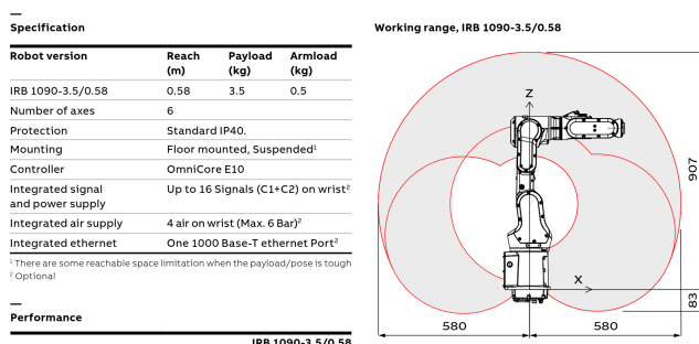
Figura 1: Especificaciones técnicas del robot
