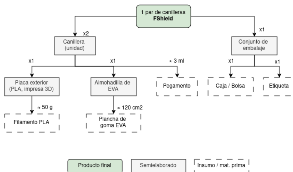
Figura 4: Diagrama de explosión y despiece (Gozinto) para un par de canilleras FShield.
