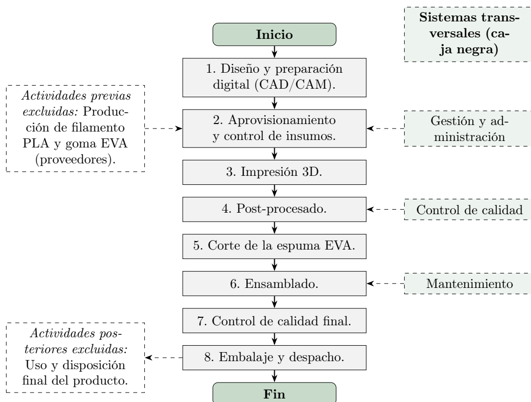
Figura 2: Diagrama de flujo del proceso productivo de FShield.
