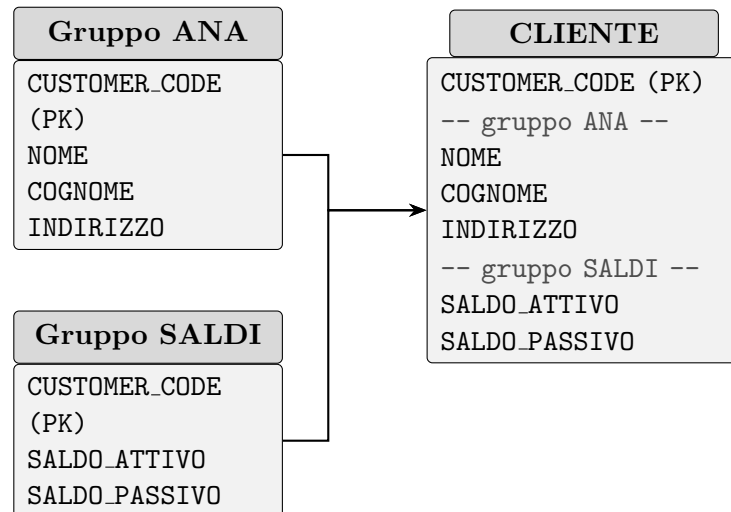
Figure 4.3: Esempio di record composito: due gruppi sorgente uniti sulla stessa chiave primaria.
