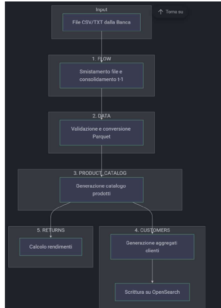
Figure 3.4: Pipeline giornaliera.
