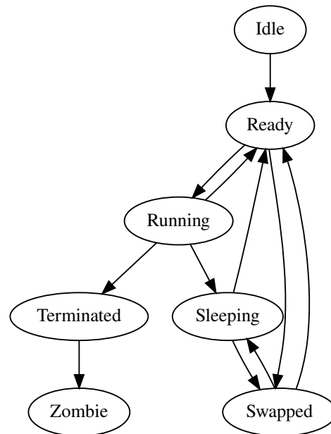
Figura 1.2: Grafo Diretto raffigurante le possibili Transizioni tra i possibili Stati di un Processo in UNIX. Grafo Generato tramite l'ausilio dell'editor PlantText[5].
