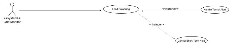
Figura 2.1: Diagramma dei casi d'uso
