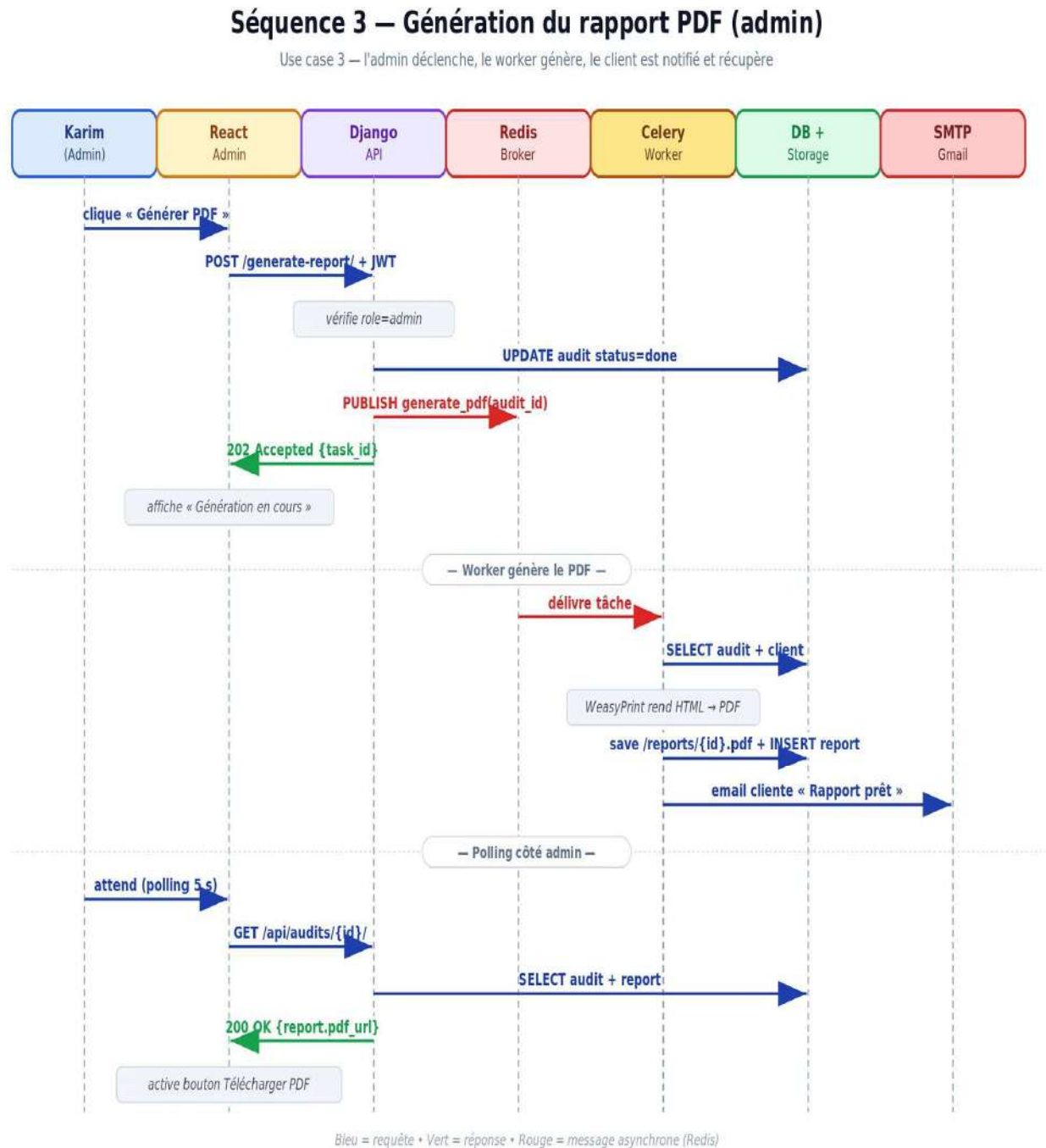
Figure 7 — Séquence Génération du rapport PDF
