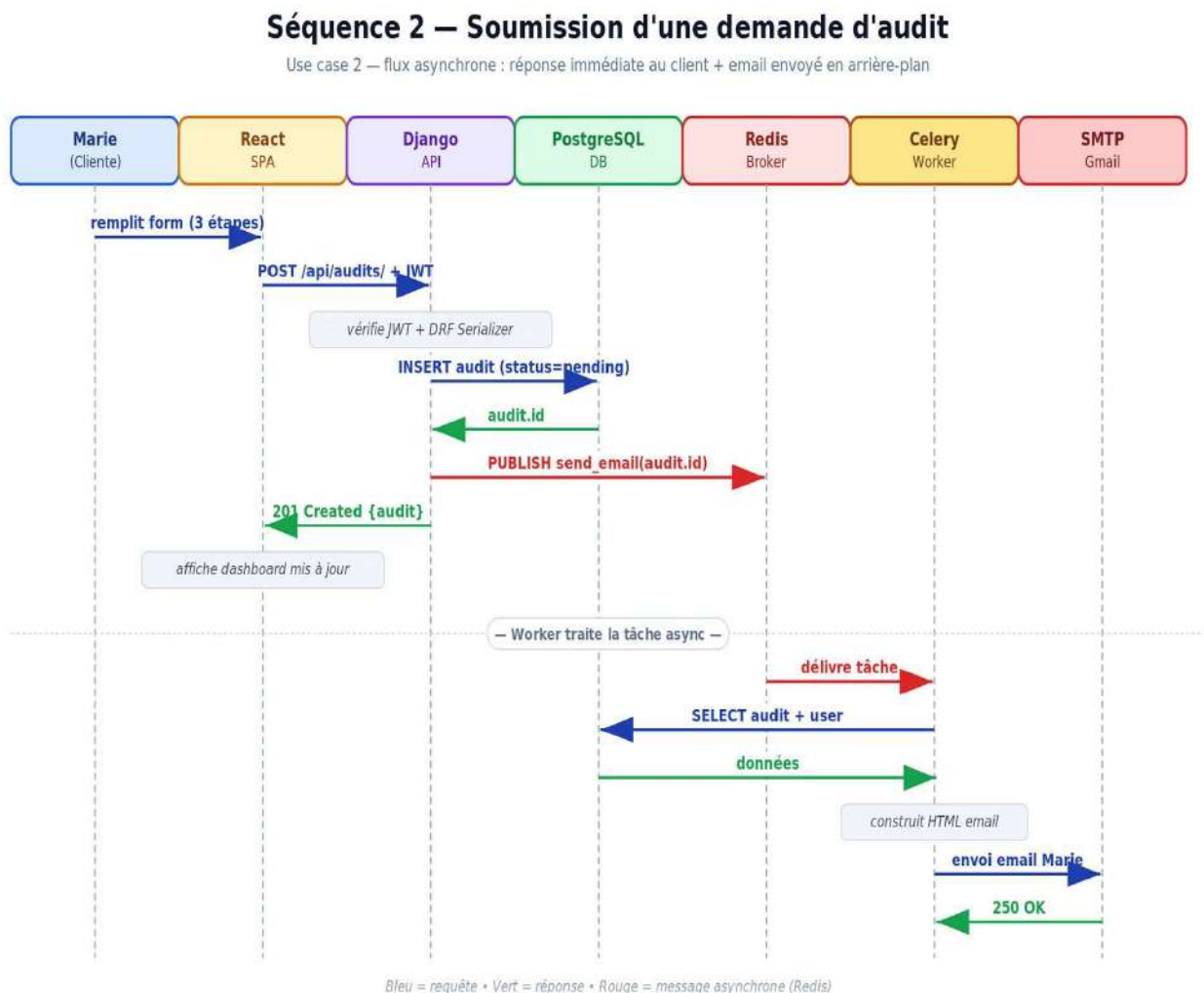
Figure 6 — Séquence Soumission demande (asynchrone Celery)
