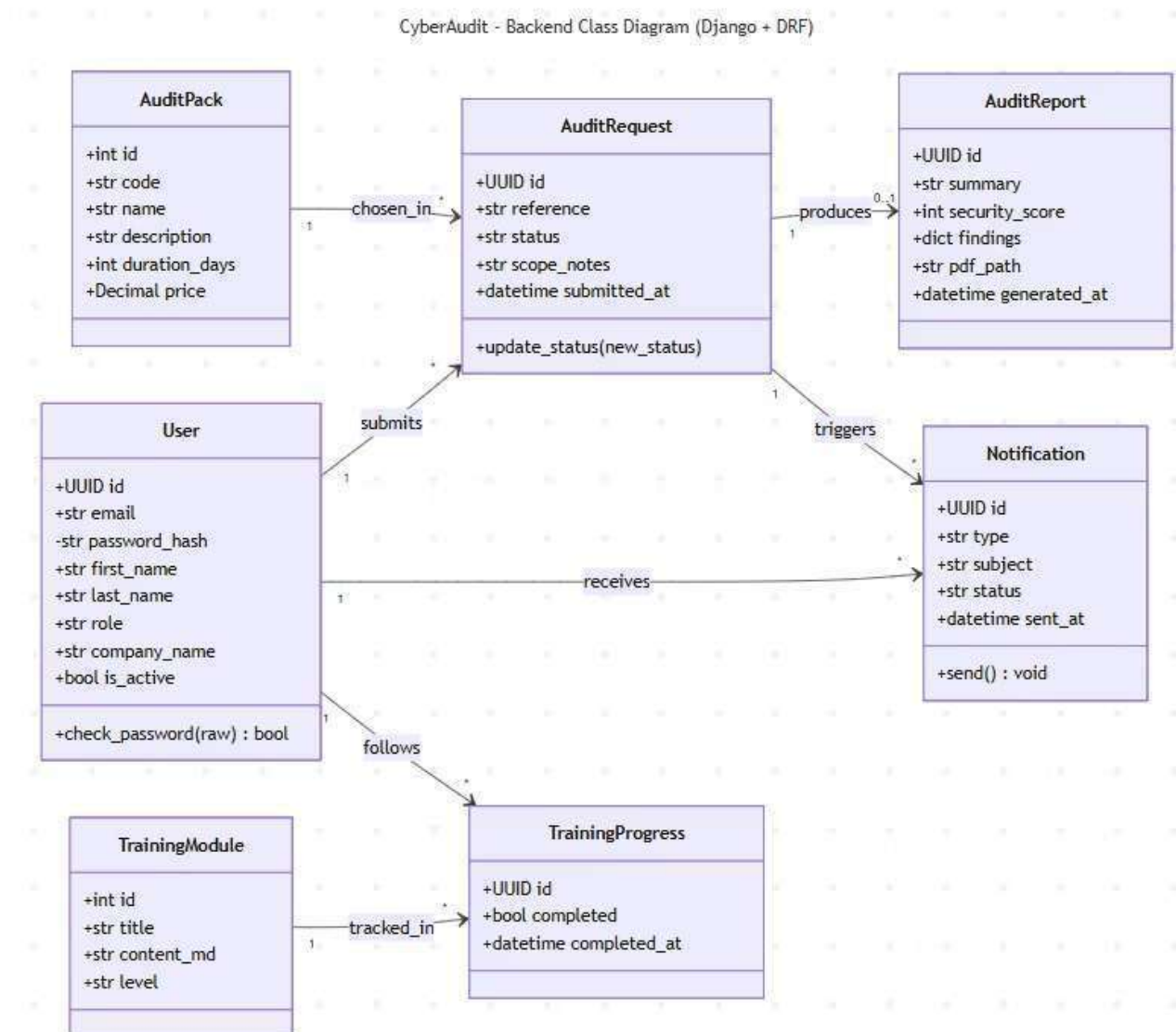
Figure 3 : Diagramme de classes back-end Django
