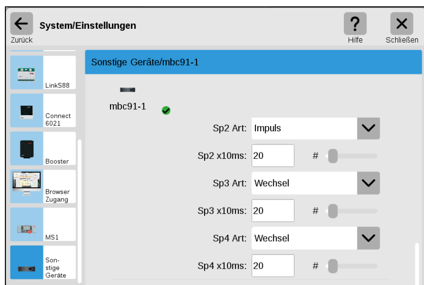
Abbildung 7-6: &lt;Einstellungen&gt;-Bereich, Teil 3
