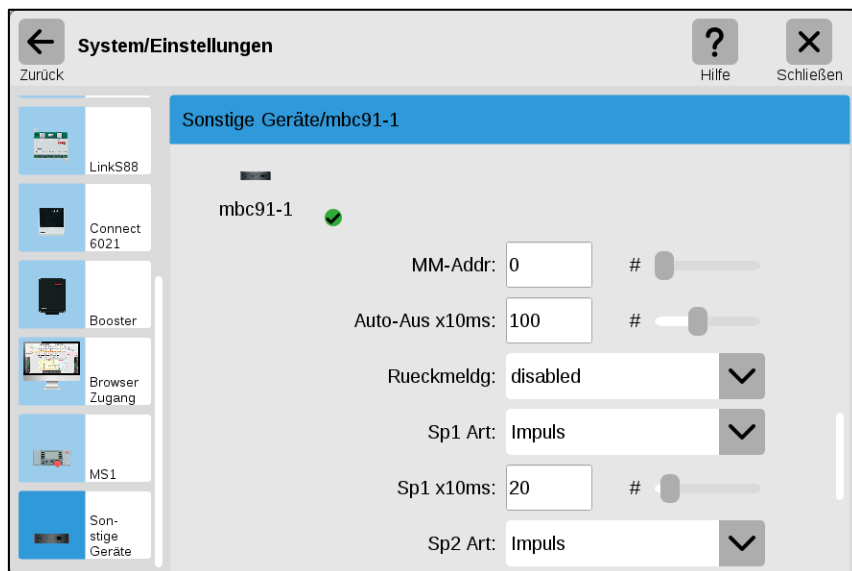
Abbildung 7-5: &lt;Einstellungen&gt;-Bereich, Teil 2
