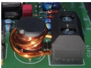
Abbildung 10-2: Übertrager
