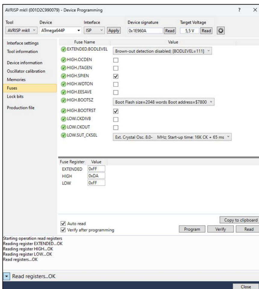
Abbildung 9-1: FUSES im AVR Studio
