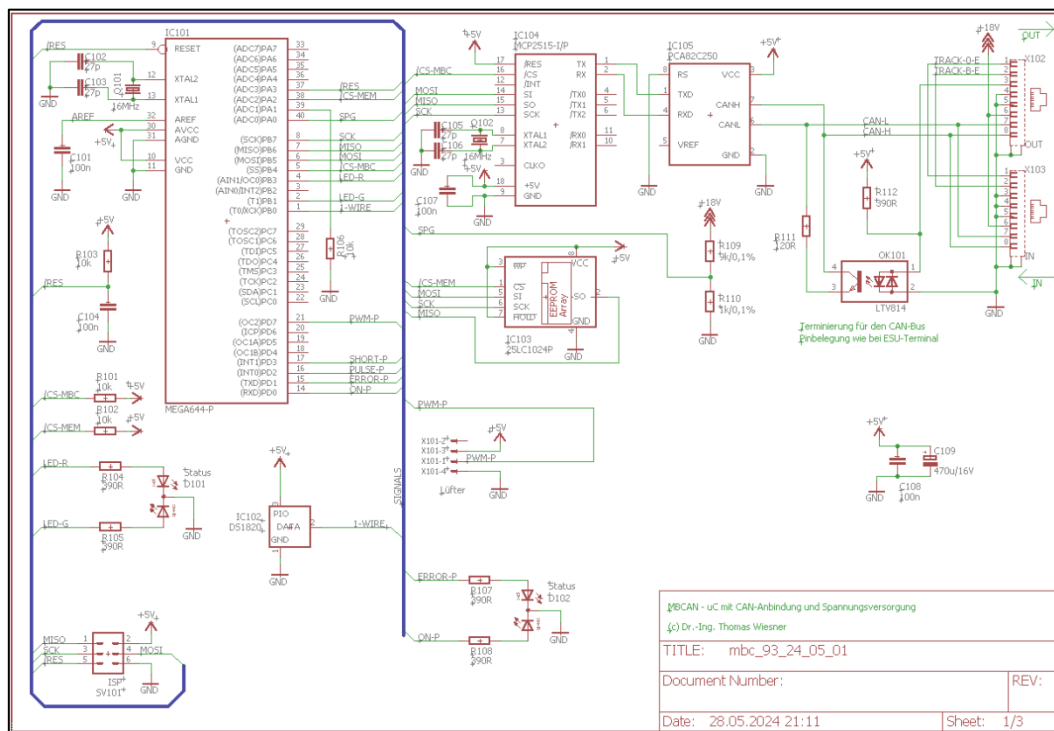
Abbildung 6-1: Schaltbild Seite 1
