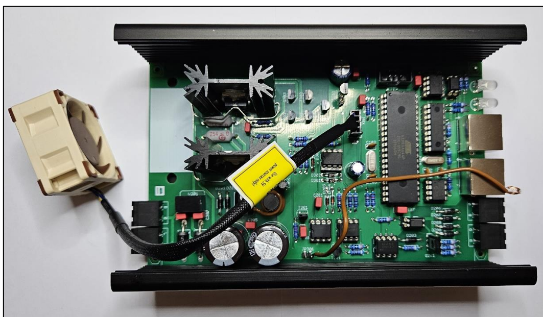
Abbildung 13-2: Bestückte Platine mit Lüfter und Gehäusepotenzialkabel
