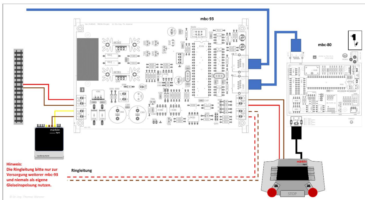
Abbildung 11-2: Anschluss an CS2 ®
