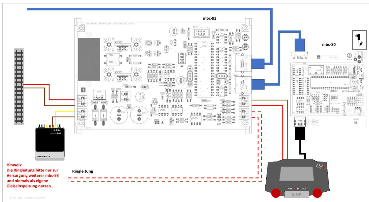
Abbildung 11-1: Anschluss an CS3 ®
