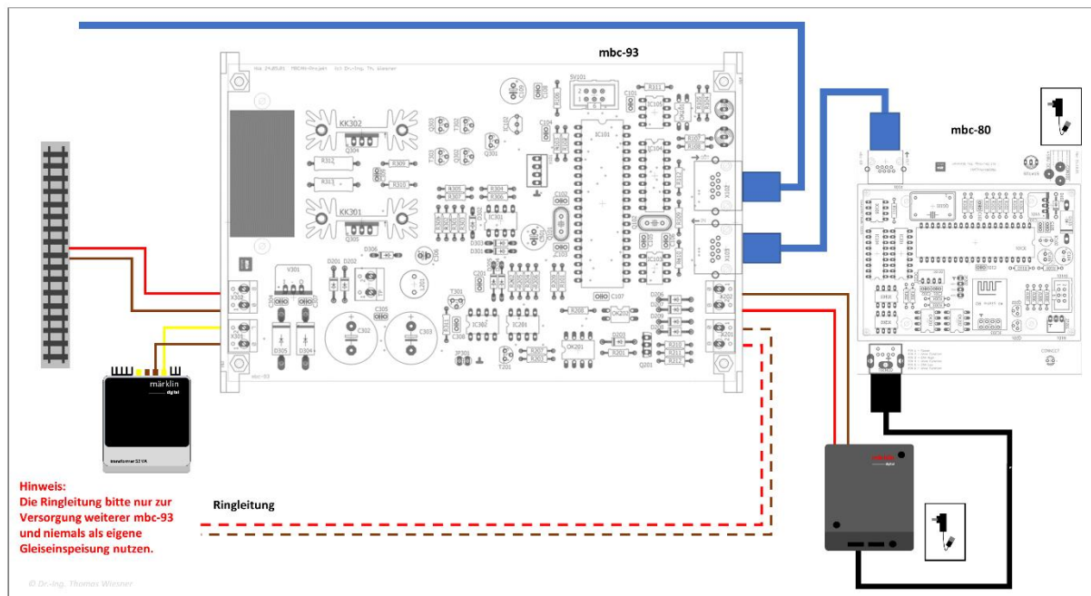
Abbildung 11-3: Anschluss an MS2®
