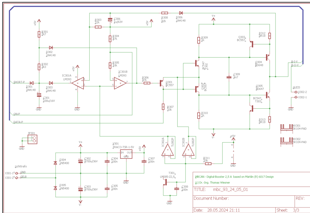
Abbildung 6-3: Schaltbild Seite 3
