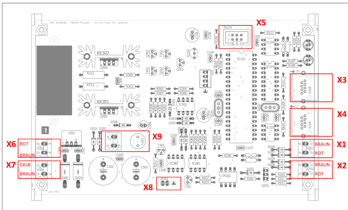
Abbildung 10-1: Steckverbinder
