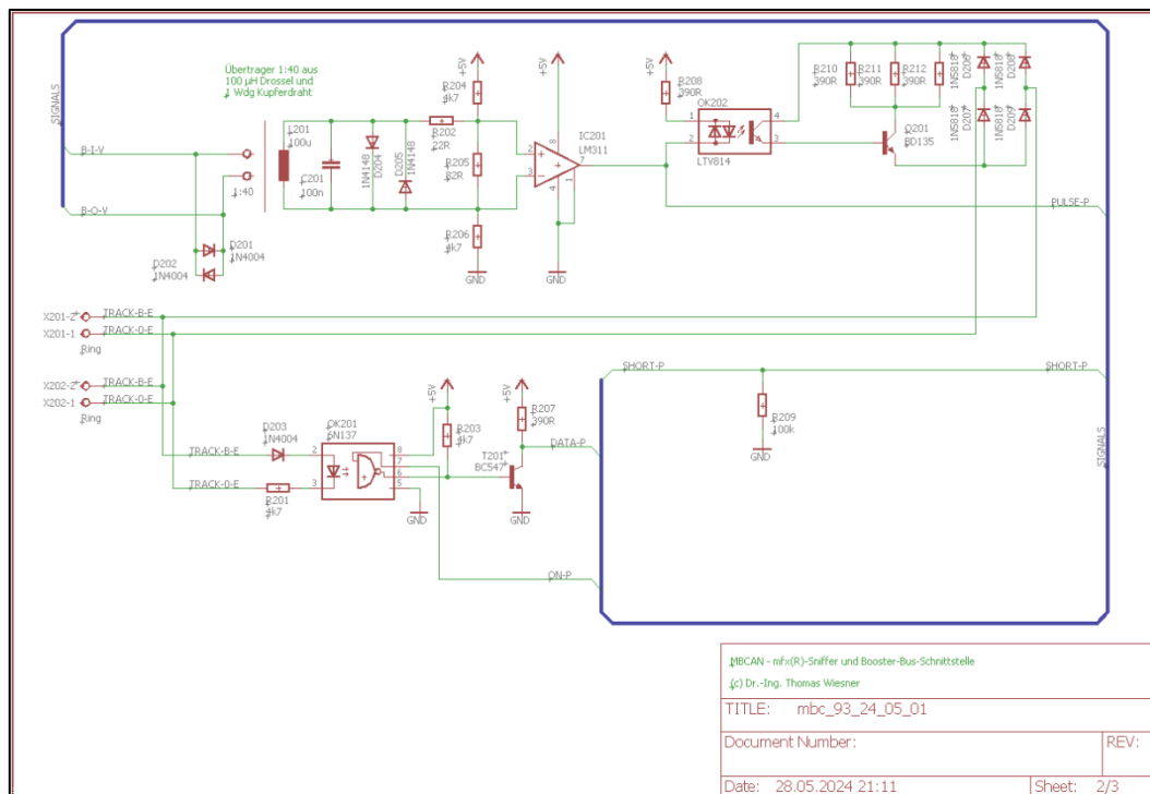
Abbildung 6-2: Schaltbild Seite 2
