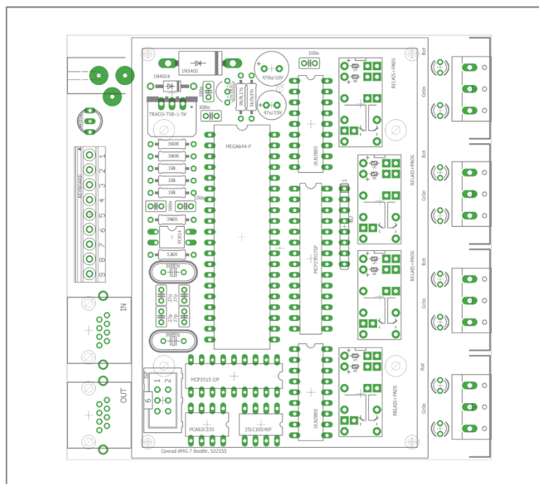
Abbildung 7-2: Bestückung Bauteilwert
