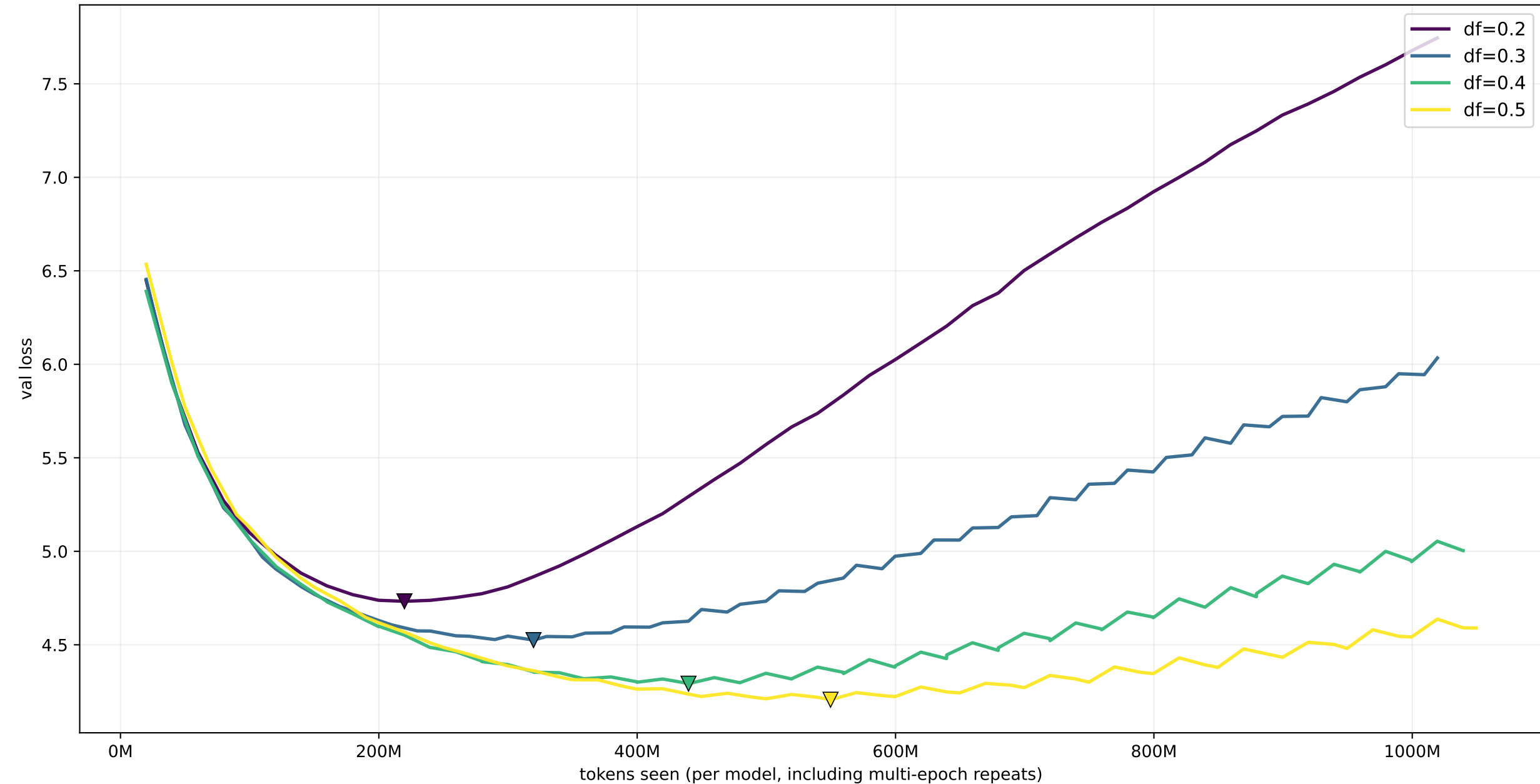
Q1: data-size ablation at d12/w768 | val resolution = 20M tokens | tag q1v2_20260503_115259
