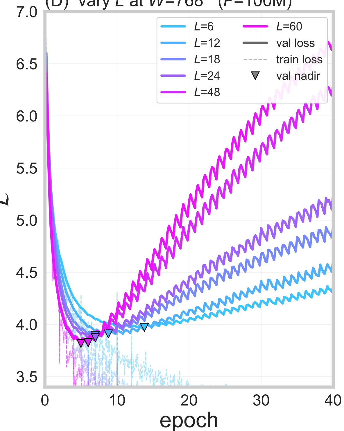
(D) vary L at W=768 ( P=100M )
