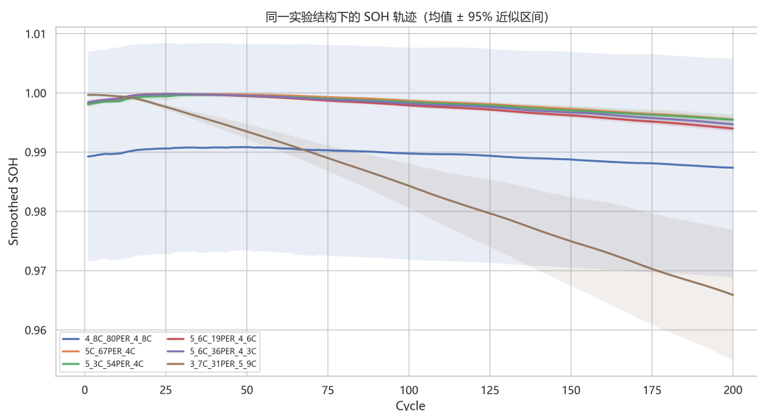
图 7 各策略的平滑 SOH 平均轨迹；阴影为均值的 95% 近似区间
