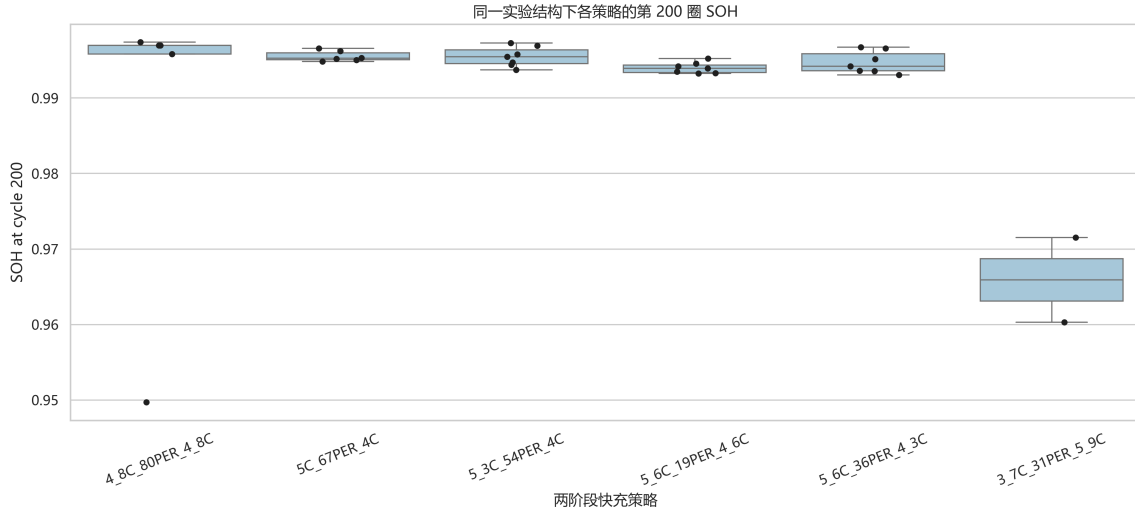
图 6 同一实验结构下，各策略第 200 圈 SOH 的箱线图与单体观测值
