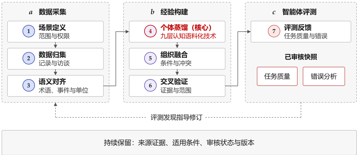
图 2 老师傅的七步流程，按数据采集、经验构建和智能体评测分组。实线箭头表示处理顺序，虚线回路将评测发现的问题反馈至语料修订。每一阶段均保留来源引用、适用条件、审核状态和版本标识。
