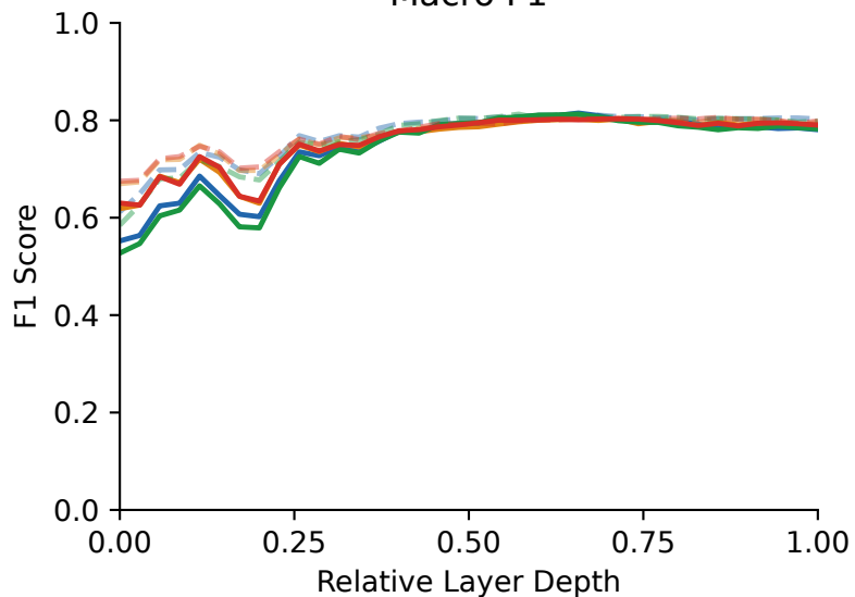
Macro F1
