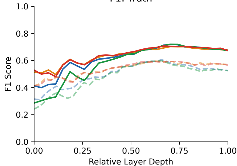
F1: Truth
