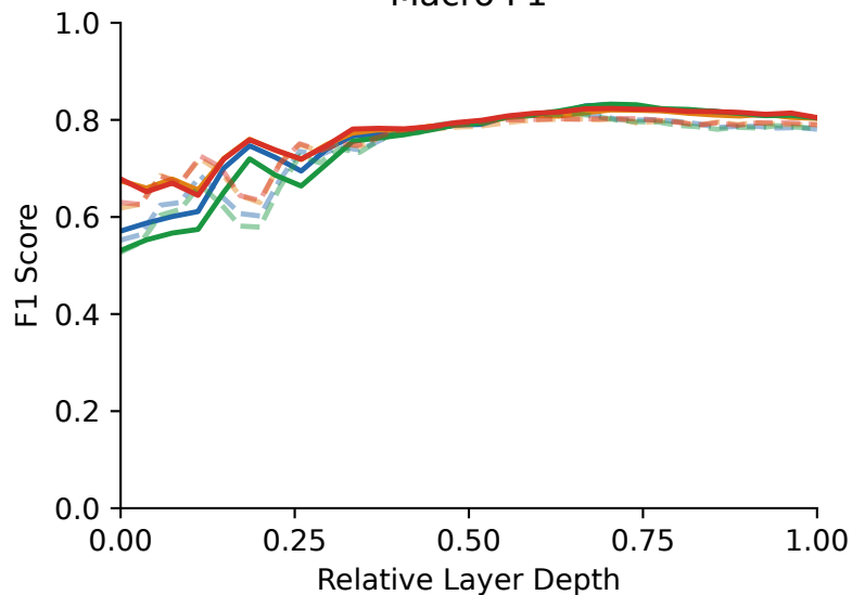
Macro F1
