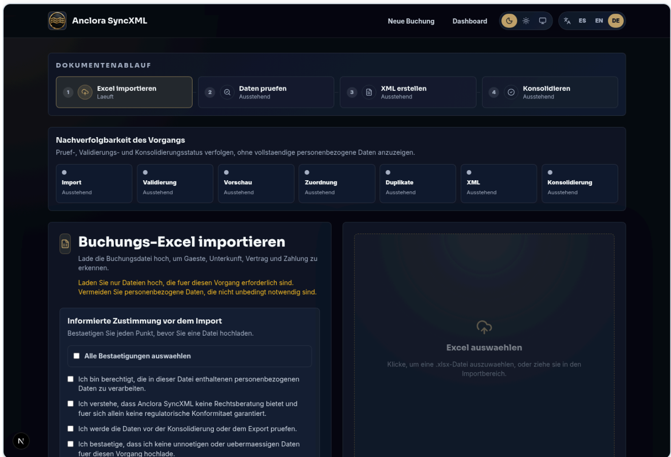
Importbildschirm
