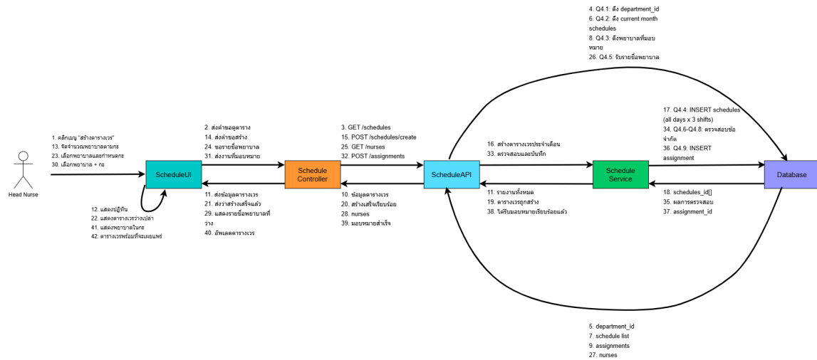
รูปที่ 4-8 Collaboration diagram ของ Use Case ที่ 4 : ออกแบบตารางเวรเบื้องต้น
