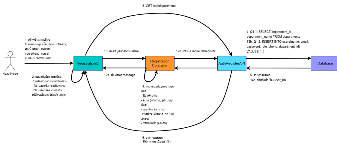
รูปที่ 4-2 Collaboration diagram ของ Use Case ที่ 1 : ลงทะเบียนผู้ใช้งานใหม่
