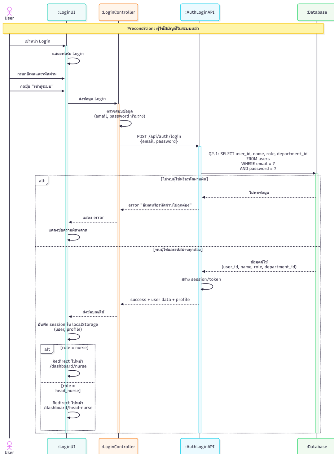
รูปที่ 4-3 Sequence Diagram ของ Use Case ที่ 2 : เข้าสู่ระบบ
