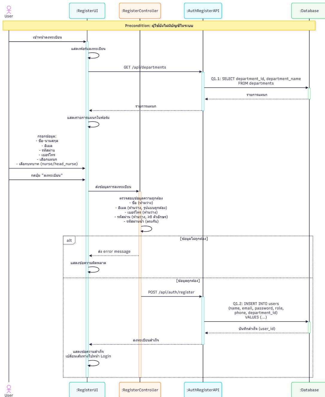
รูปที่ 4-1 Sequence Diagram ของ Use Case ที่ 1 : ลงทะเบียนผู้ใช้งานใหม่
