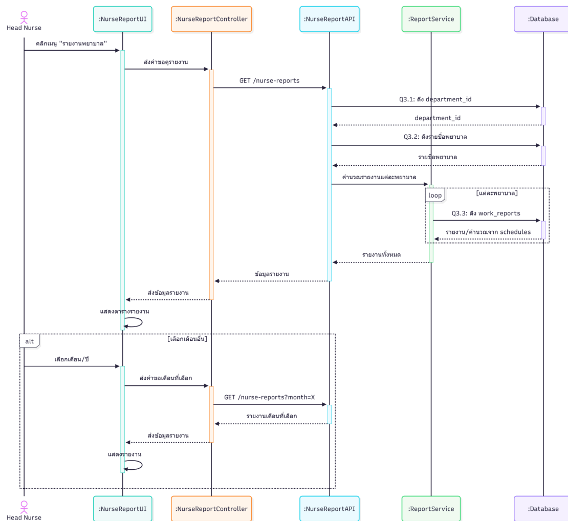
รูปที่ 4-5 Sequence Diagram ของ Use Case ที่ 3 : วิเคราะห์ความต้องการจาก report รายเดือน
