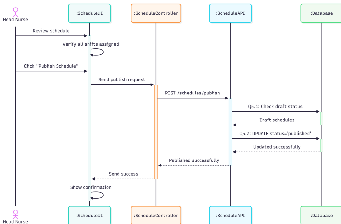
รูปที่ 4-9 Sequence Diagram ของ Use Case ที่ 5 : กดประกาศเวร
