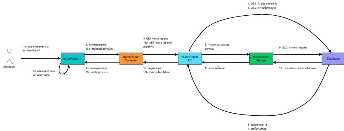
รูปที่ 4-6 Collaboration diagram ของ Use Case ที่ 3 : วิเคราะห์ความต้องการจาก report รายเดือน
