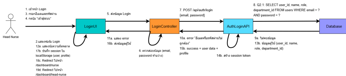
รูปที่ 4-4 Collaboration diagram ของ Use Case ที่ 2 : เข้าสู่ระบบ
