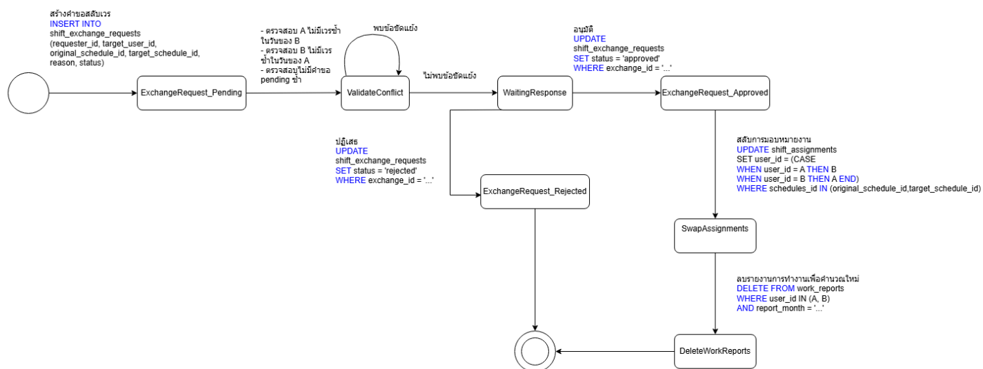
รูปที่ 5-4 State Diagram ของการขอสลับเวร
