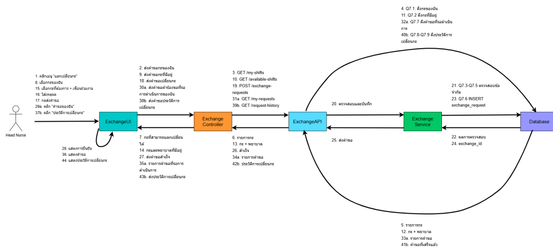
รูปที่ 4-14 Collaboration Diagram ของ Use Case ที่ 7 : ส่งคำขอแลกเวร
