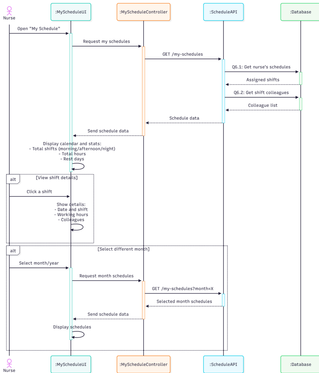
รูปที่ 4-11 Sequence Diagram ของ Use Case ที่ 6 : ตรวจสอบตารางเวร
