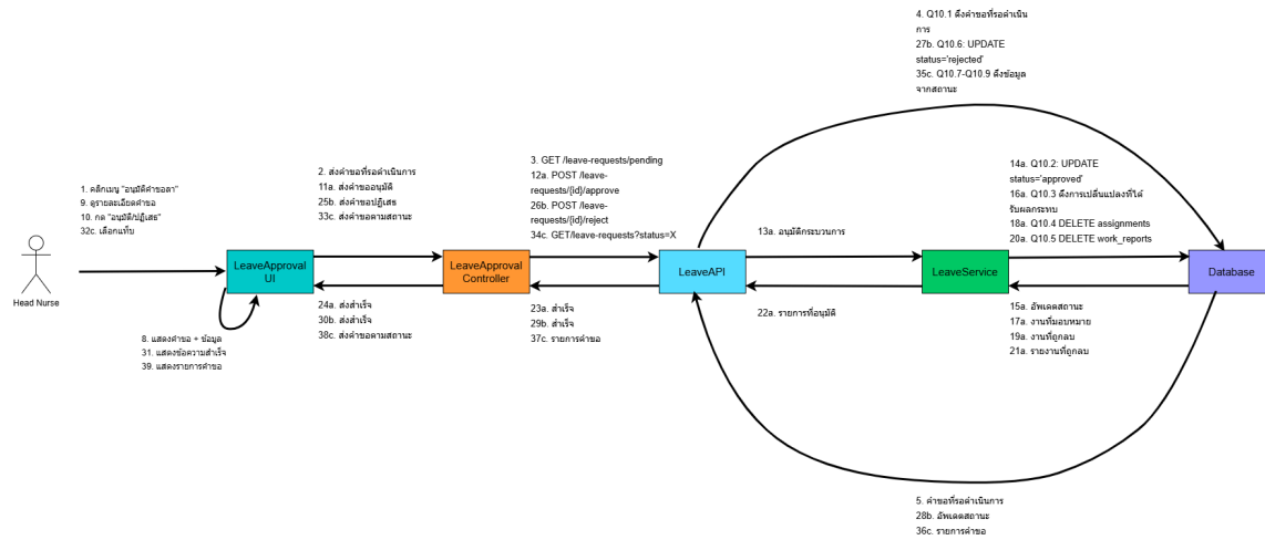
รูปที่ 4-20 Collaboration Diagram ของ Use Case ที่ 10 : อนุมัติ/ปฏิเสธ การลา
