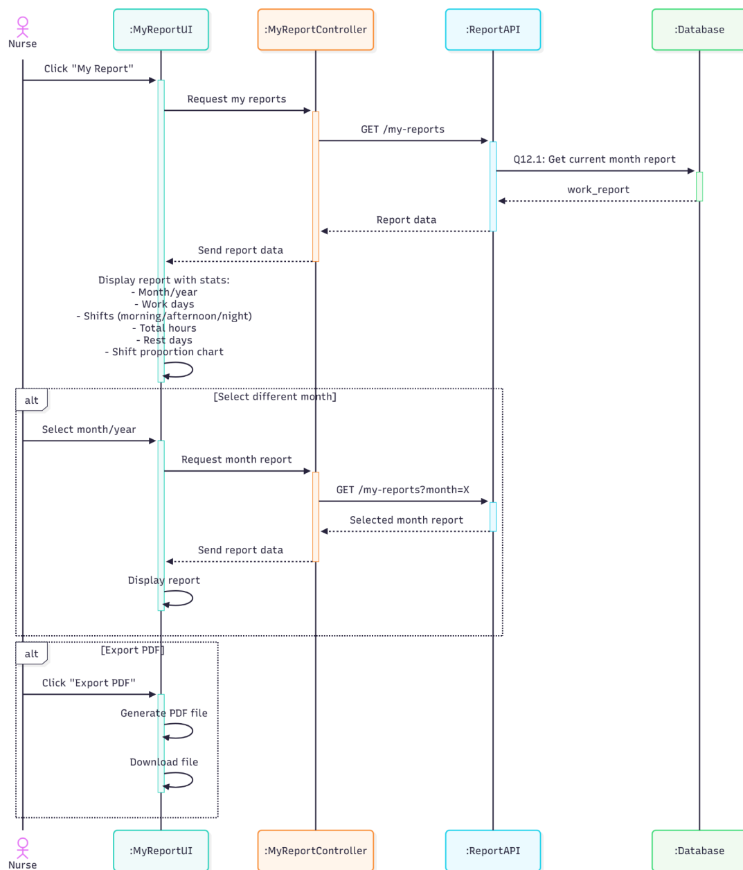
รูปที่ 4-23 Sequence Diagram ของ Use Case ที่ 12 : รายงานของพยาบาล
