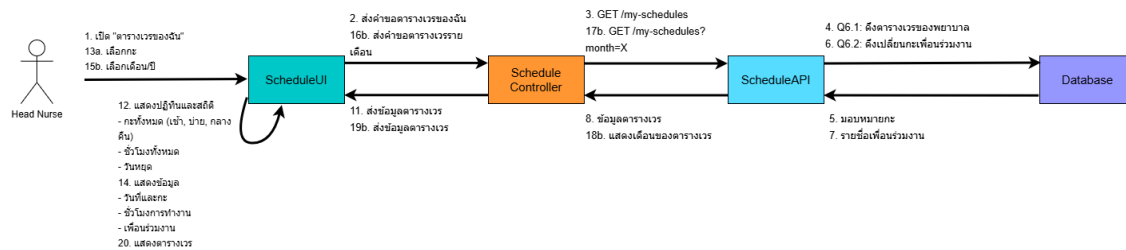
รูปที่ 4-12 Collaboration diagram ของ Use Case ที่ 6 : ตรวจสอบตารางเวร
