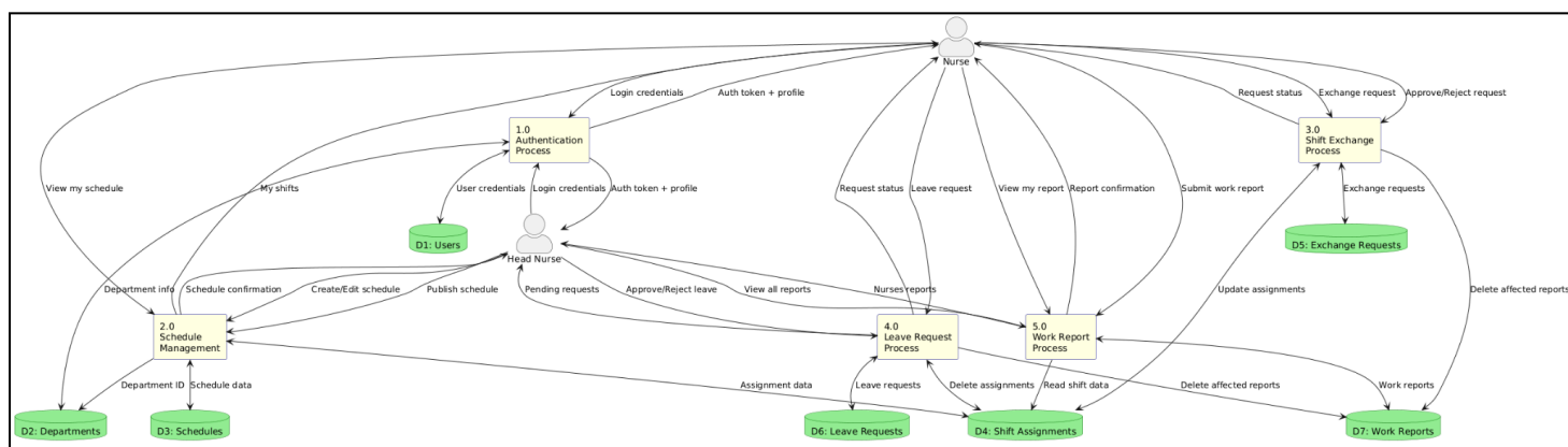
รูปที่ 5-7 Data flow diagram Level-1 (Major Processes)
