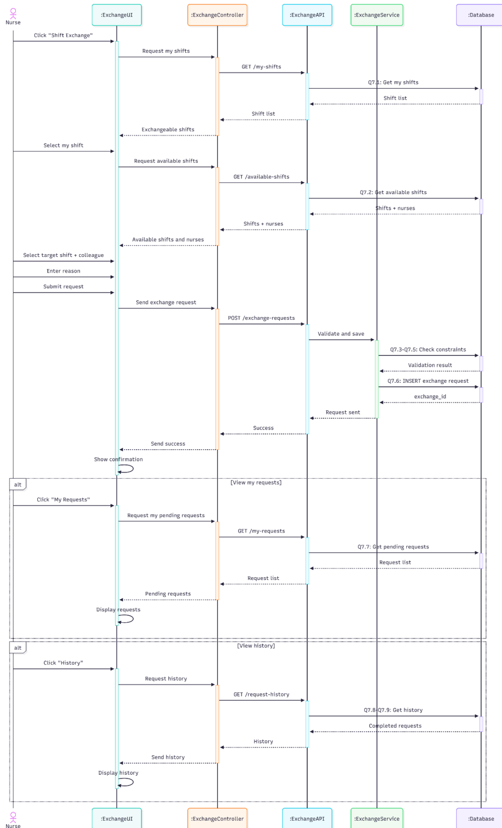
รูปที่ 4-13 Sequence Diagram ของ Use Case ที่ 7 : ส่งคำขอแลกเวร
