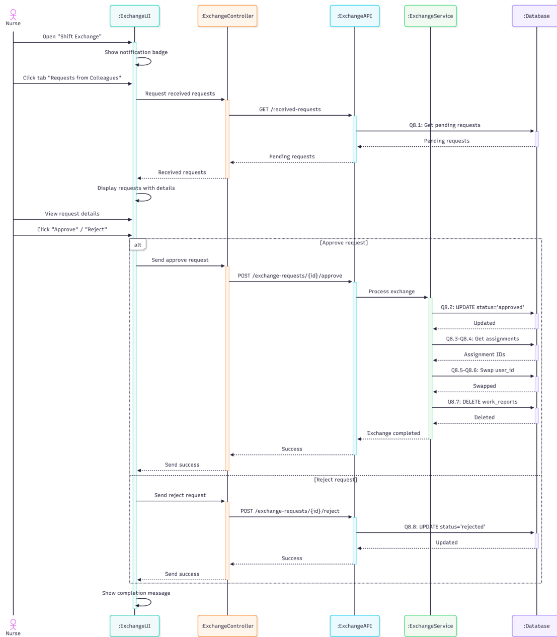
รูปที่ 4-15 Sequence Diagram ของ Use Case ที่ 8 : อนุมัติ/ปฏิเสธ การแลกเวร
