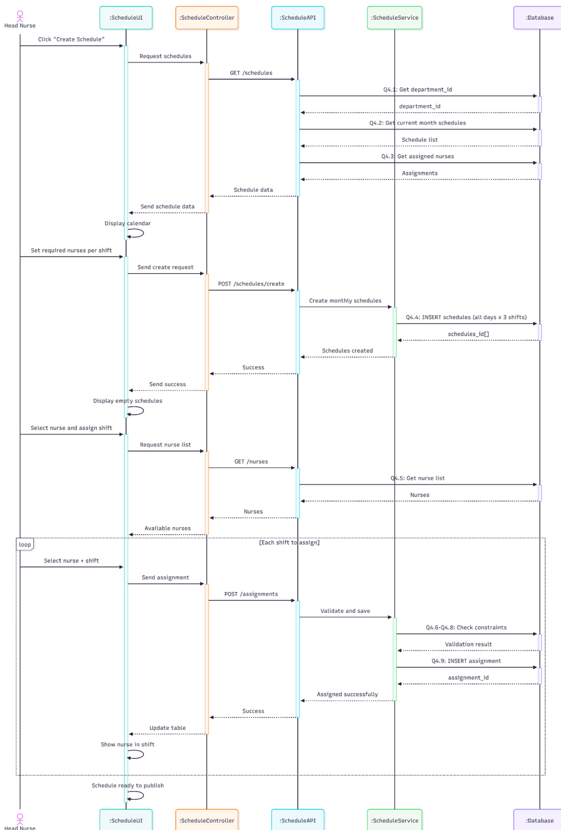
รูปที่ 4-7 Sequence Diagram ของ Use Case ที่ 4 : ออกแบบตารางเวรเบื้องต้น
