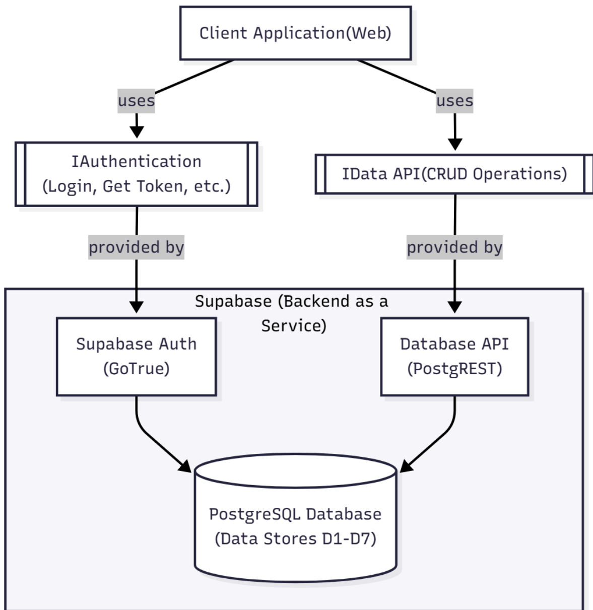
รูปที่ 5-8 Component Diagram
