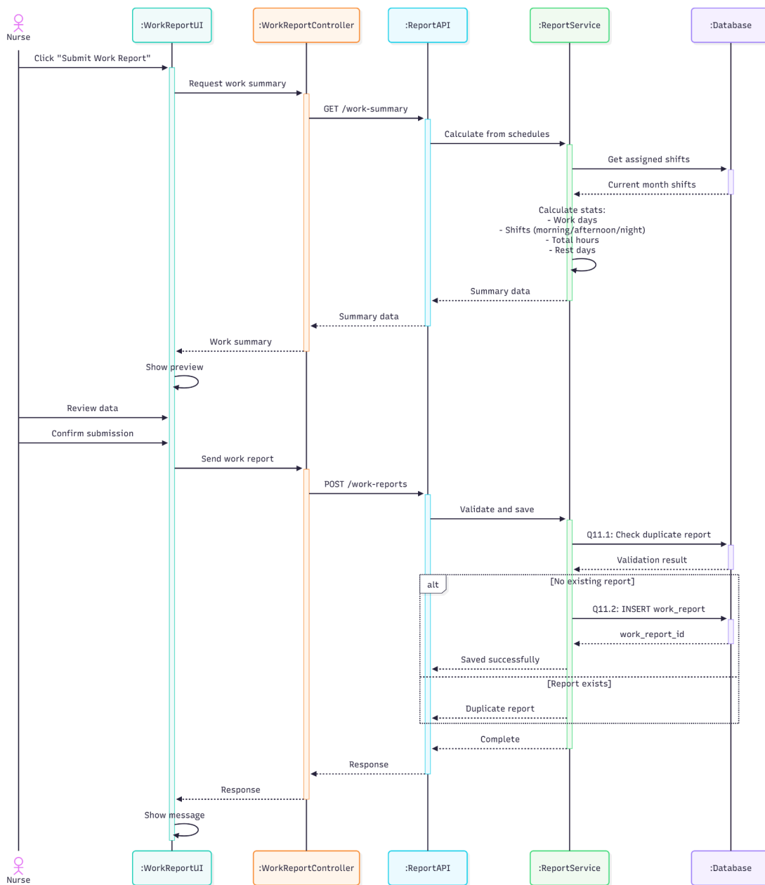
รูปที่ 4-21 Sequence Diagram ของ Use Case ที่ 11 : บันทึกการทำงานตามตารางเวรของพยาบาล
