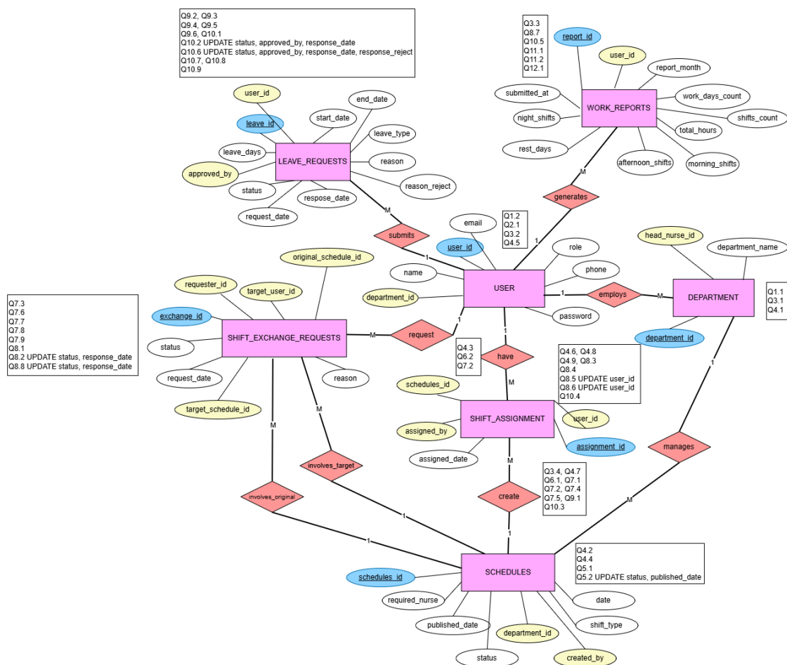
รูปที่ 5-2 แสดงข้อมูล ER Diagram ที่มี Query
