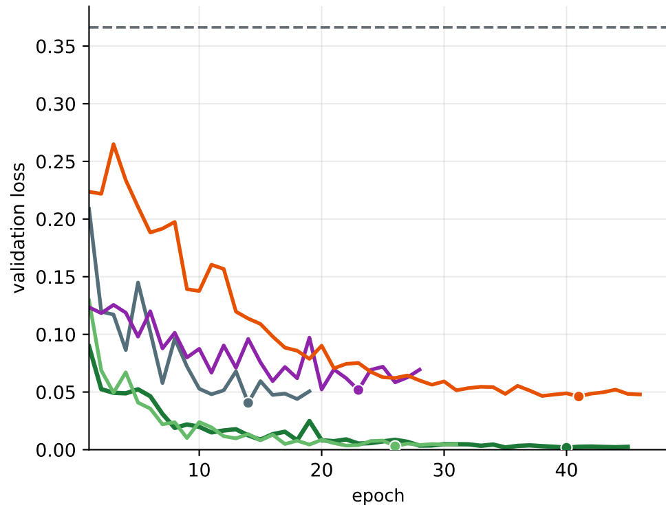
Stage-1 TSQA
