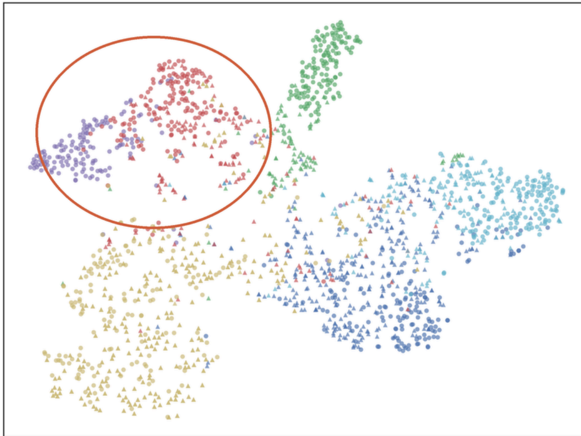
Baseline
