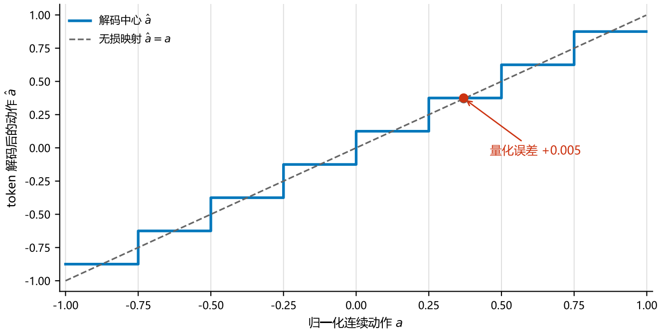
均匀动作 token: 分箱、中心解码与量化误差
