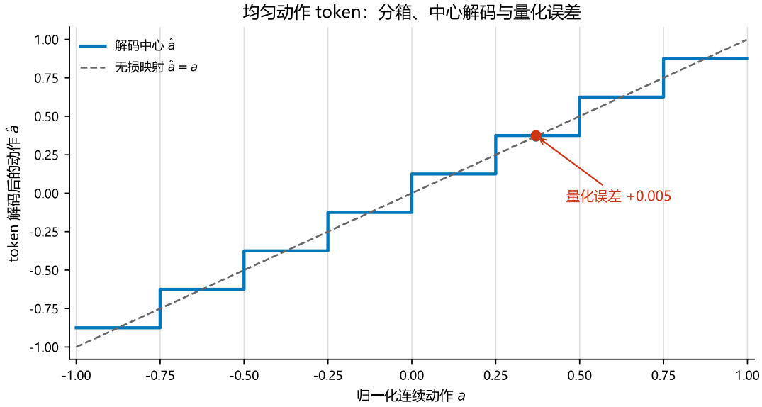
图 2.3: 均匀动作分箱的阶梯解码与误差。作者依据 OpenVLA 的动作 tokenizer 逻辑绘制 [14-15] ；图中使用 B = 8 仅为放大展示量化效应。
