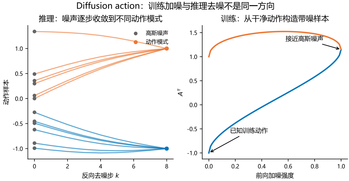
图 2.4: 扩散动作的训练加噪与推理去噪方向。作者根据 Diffusion Policy 的方法与原论文 Fig. 1、Fig. 3 重新组织绘制 [9] ，不复制原像素；轨迹为教学示意。
