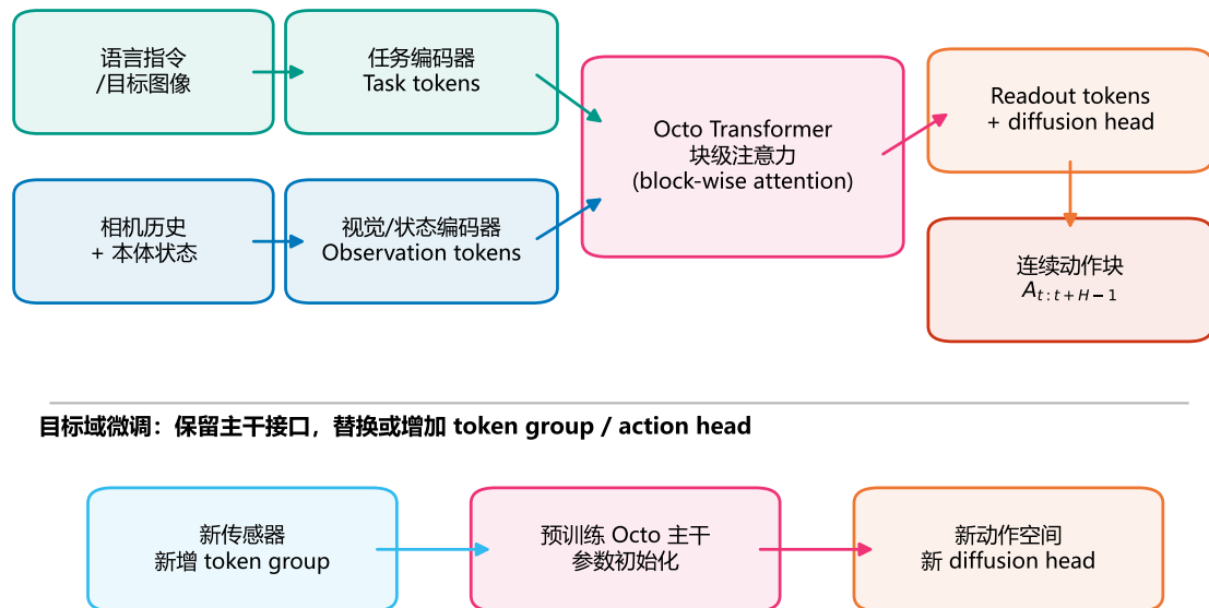
图 2.6: Octo 的模块化输入、Transformer 主干、readout 与动作头，以及目标域新增接口。作者依据 Octo 原论文 Fig. 2 改绘 [10] ，不复制原图像素。
