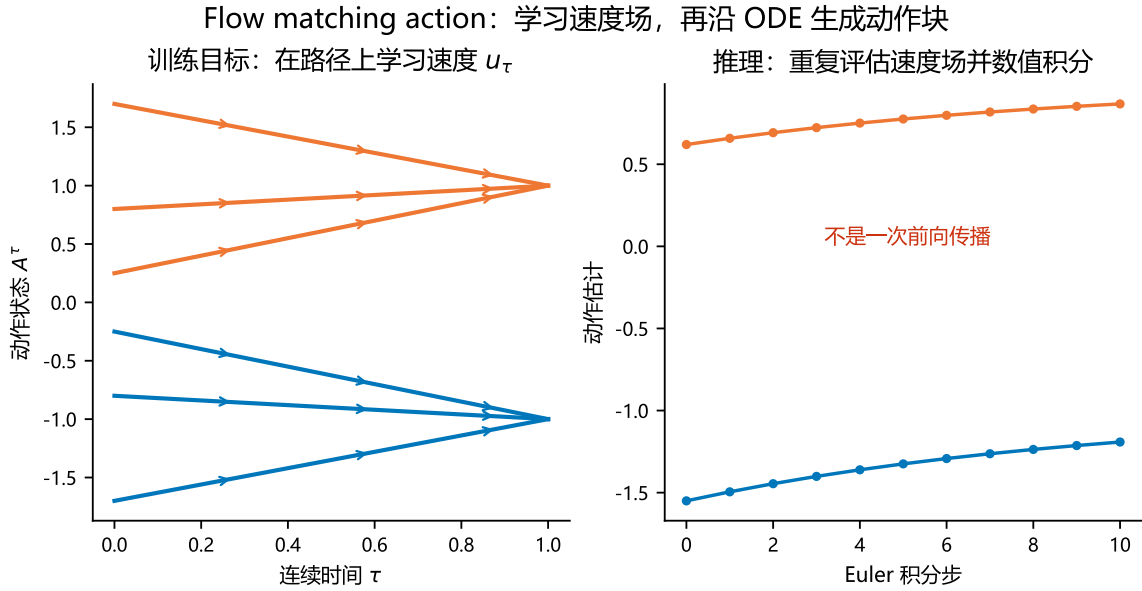
图 2.5: 流匹配的训练速度场与 Euler 推理。作者依据 \pi_0 的 flow-matching 动作专家改绘 [11] ；路径为二维教学投影。
