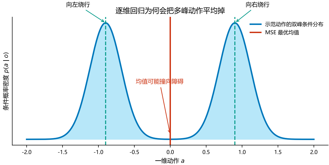
图 2.2: 平方误差把双峰动作分布压成条件均值的教学示意。曲线为作者生成的合成分布，不是论文实验结果。
