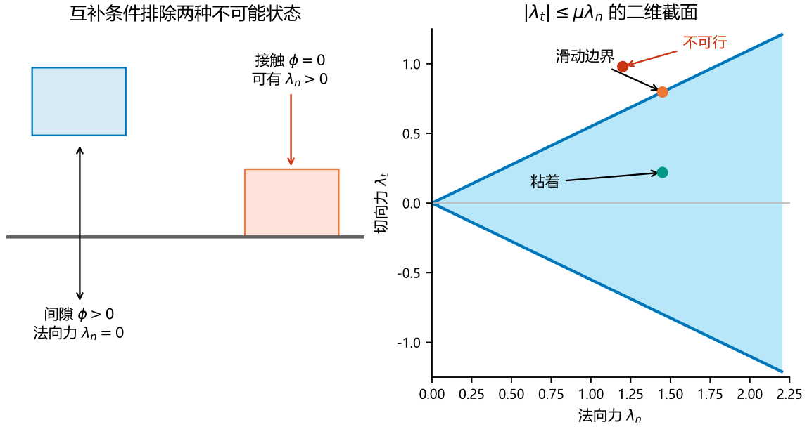
图 1.1：法向互补的合法/非法状态与库仑摩擦锥截面。作者依据刚性接触模型绘制；图为概念解释，不是实验数据 [3-4] 。
