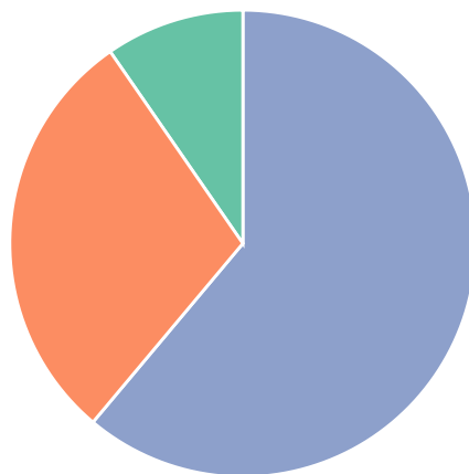
m6A
