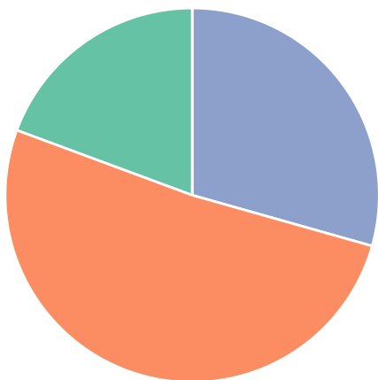
Pseudouridine (..)
