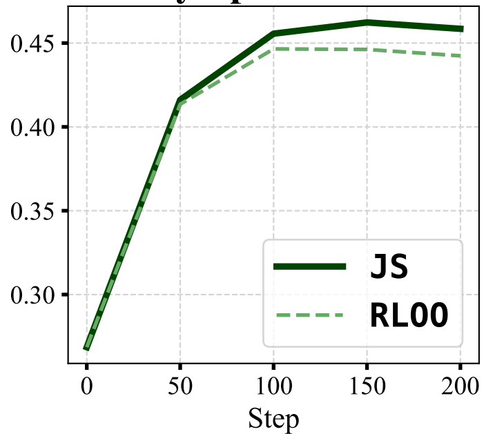
OlympiadBench
