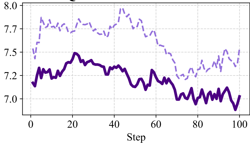
\times 10^{-5} Qwen2.5-Math-1.5B
