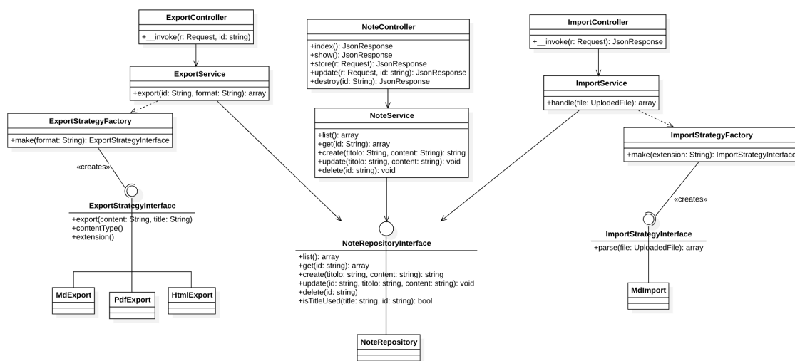
Figura 1: Diagramma delle classi per Gestione note - Esportazione - Importazione
