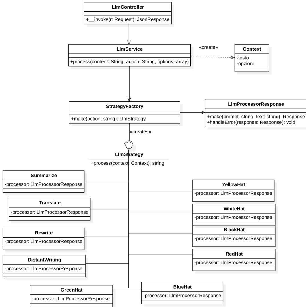
Figura 2: Diagramma delle classi per Interazione con LLM
