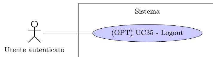
Figura 42: UC35 - Logout
