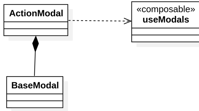
Figura 5: Diagramma UML componente ActionModal
