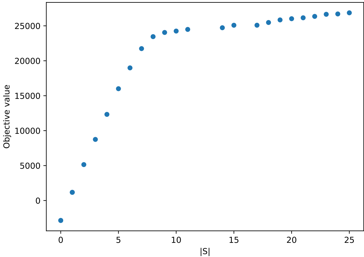
Trade-off - GSEMO_PWT - 2300
