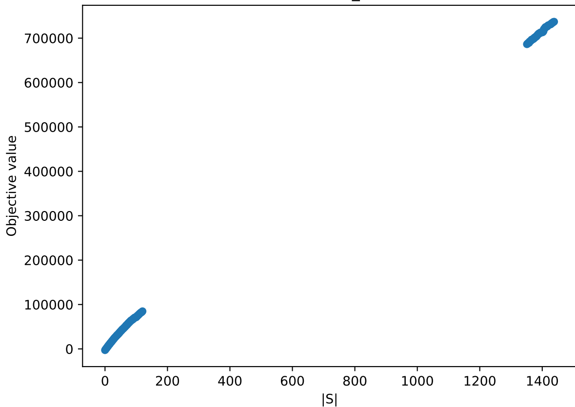
Trade-off - GSEMO_PWT - 2302
