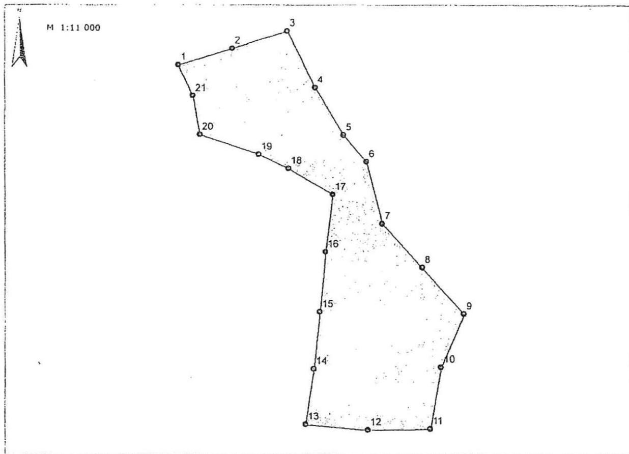
КООРДИНАТИ НА ХАРАКТЕРНИТЕ ТОЧКИ ОТ КОНТУРА НА ОБЕКТА (координатна система БГС 2005, тип на координатите - кадастрални)
