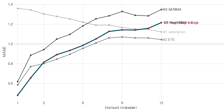
Figur 3: MASE per horisont. Stiplet linje ved 1 er sesongnaiv prognose i treningsvinduet. Ingen modell dominerer over hele horisonten: de regelinformerte er klart best på korte horisonter, mens forspranget spises opp mot tolv måneder.
