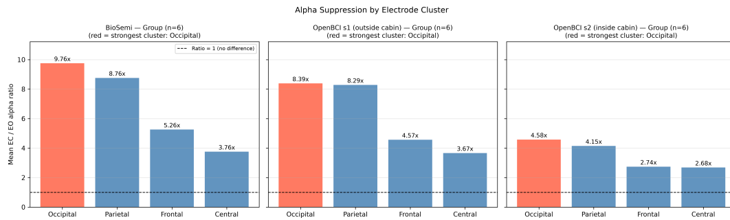
Abbildung 4.3: Alpha-Suppression an den okzipitalen Elektroden für alle drei Versuchsbedingungen
