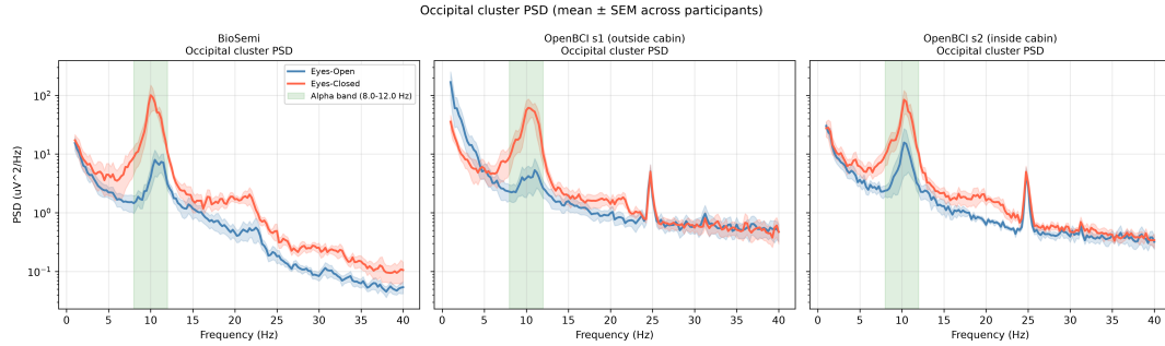
Abbildung 4.2: Ergebnis der Frequenzbandanalyse an den okzipitalen Elektroden für alle drei Versuchsbedingungen
