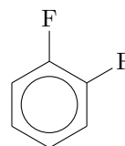
1,2-difluorobenzene
