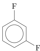
m -difluorobenzene (1,3-difluorobenzene)
