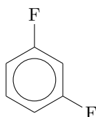
m -difluorobenzene (1,3-difluorobenzene)
