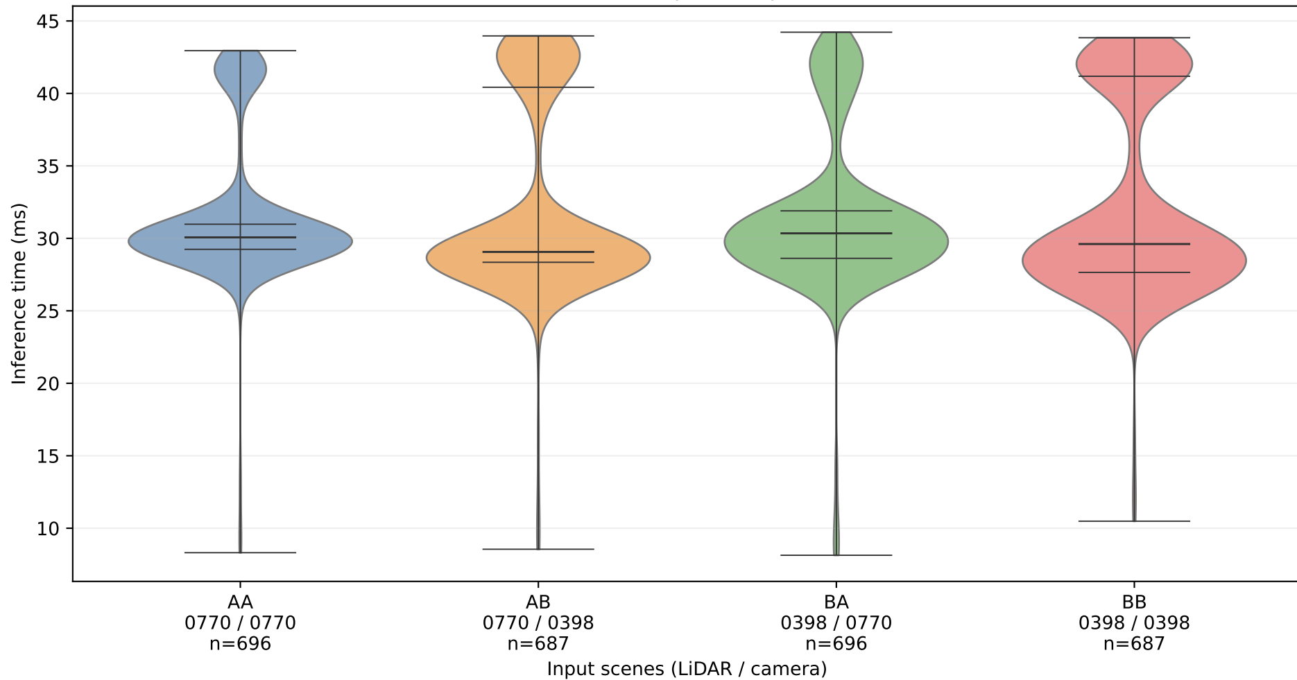
3dssd+yolov3 | yolov3 | MPS off
